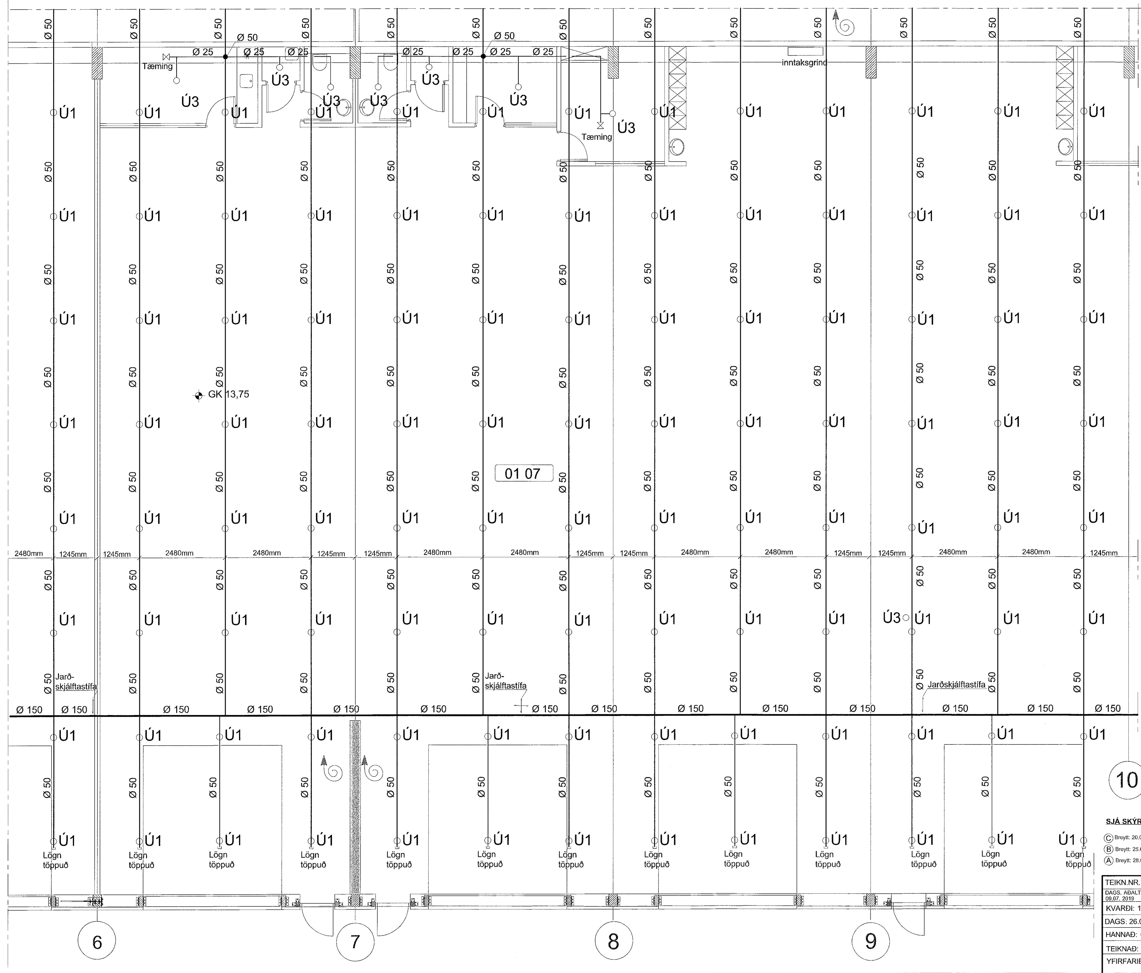
LYKILMYND 1:1000
