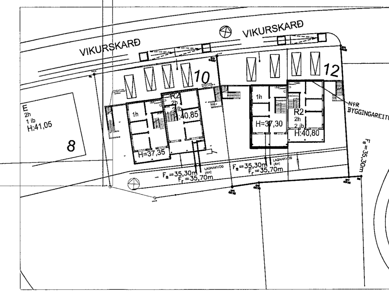
Afstöðumynd Mkv. 1:500.
