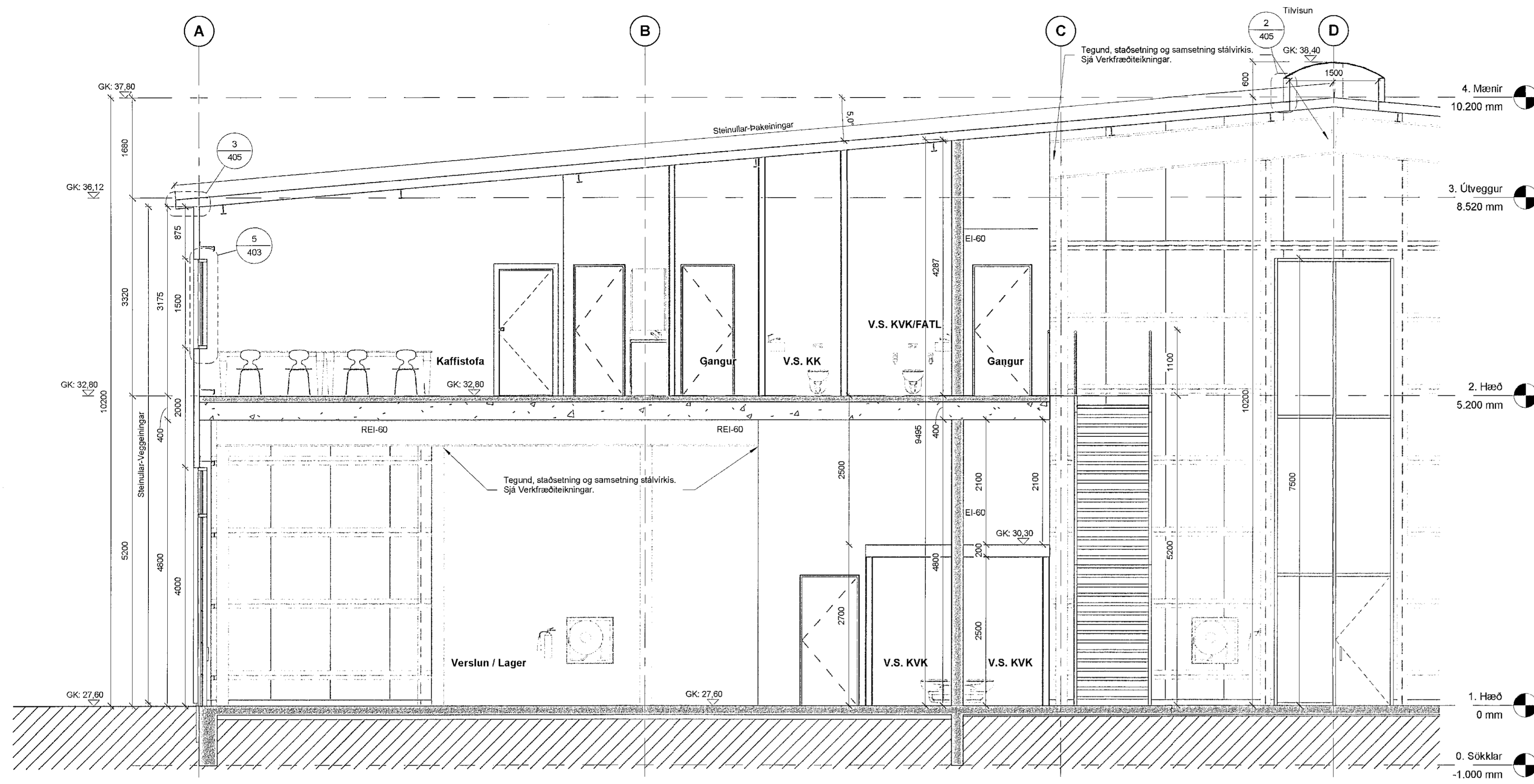
1 Snið A-A VT - Vestur 1 : 50
