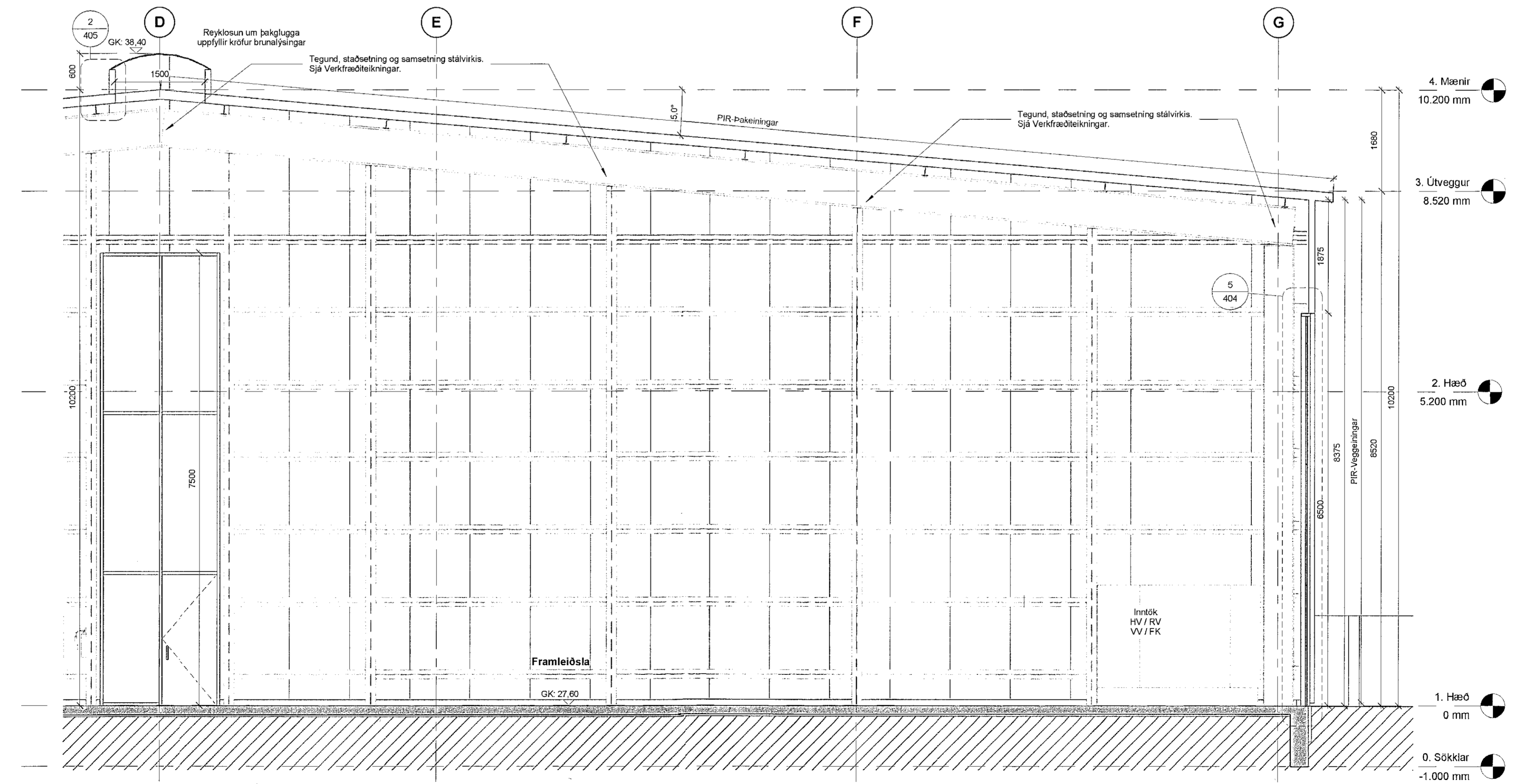
2 Snið A-A VT - Austur 1 : 50
