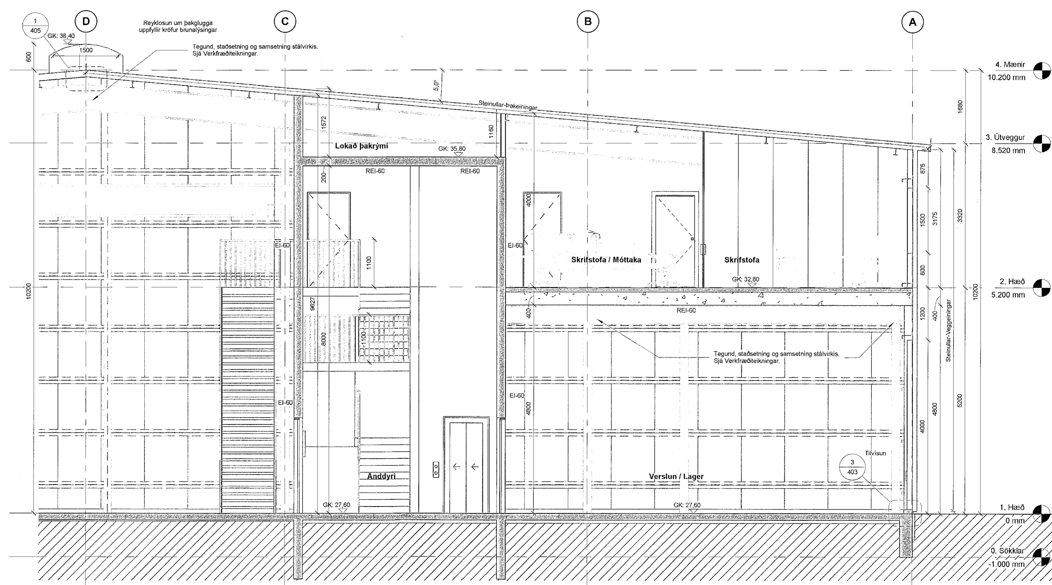
2 Snið B-B VT - Vestur 1 : 50
