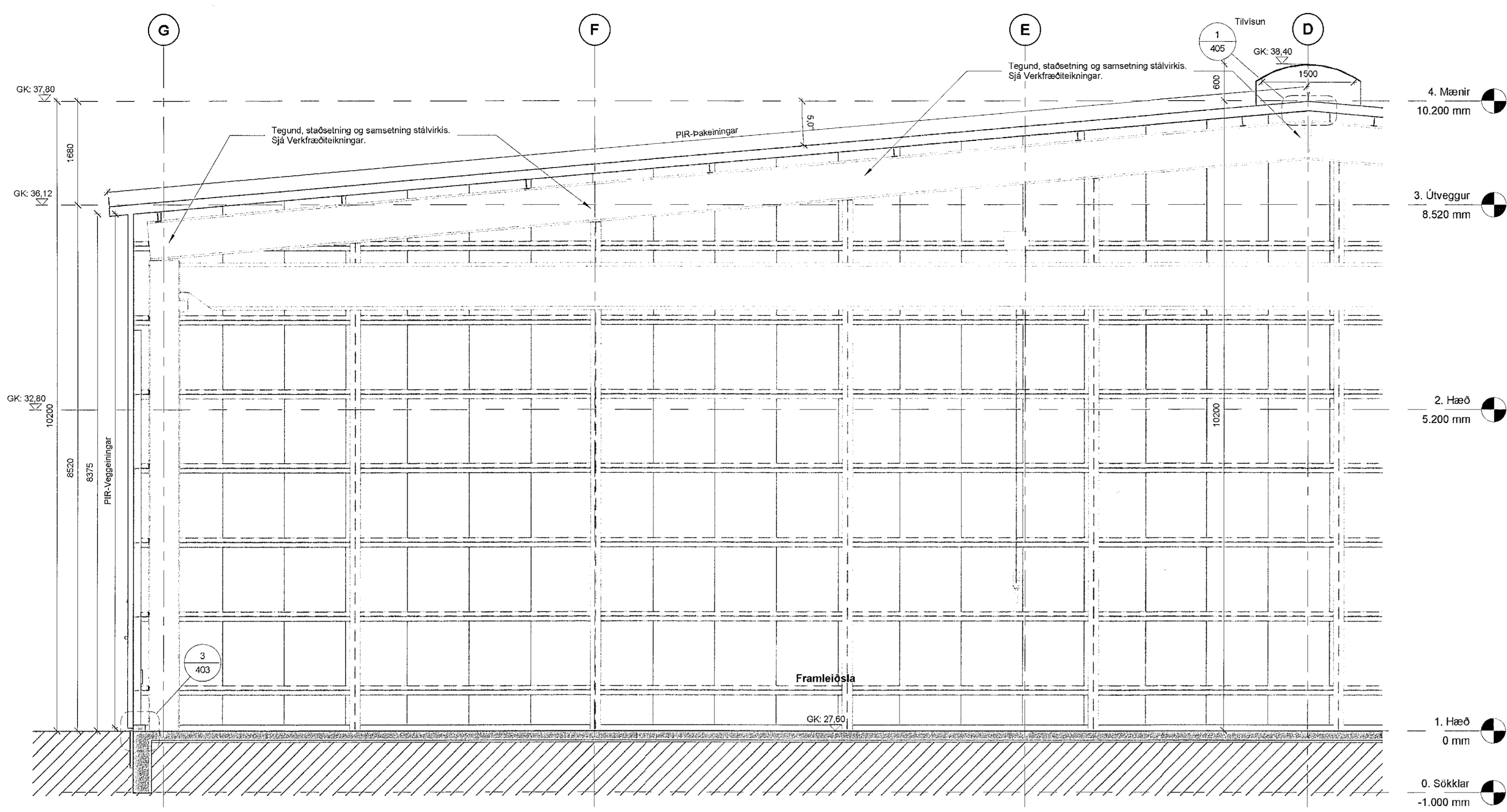
1 Snið B-B VT - Austur 1 : 50
