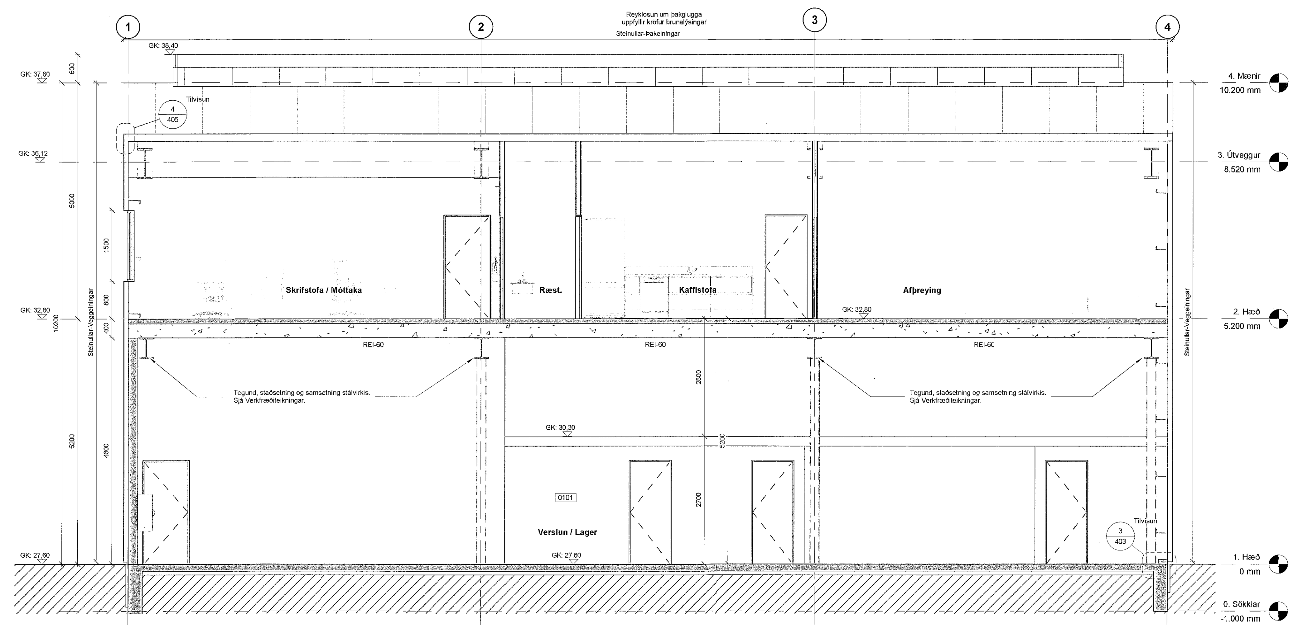
2 Snið D-D VT 1 : 50
