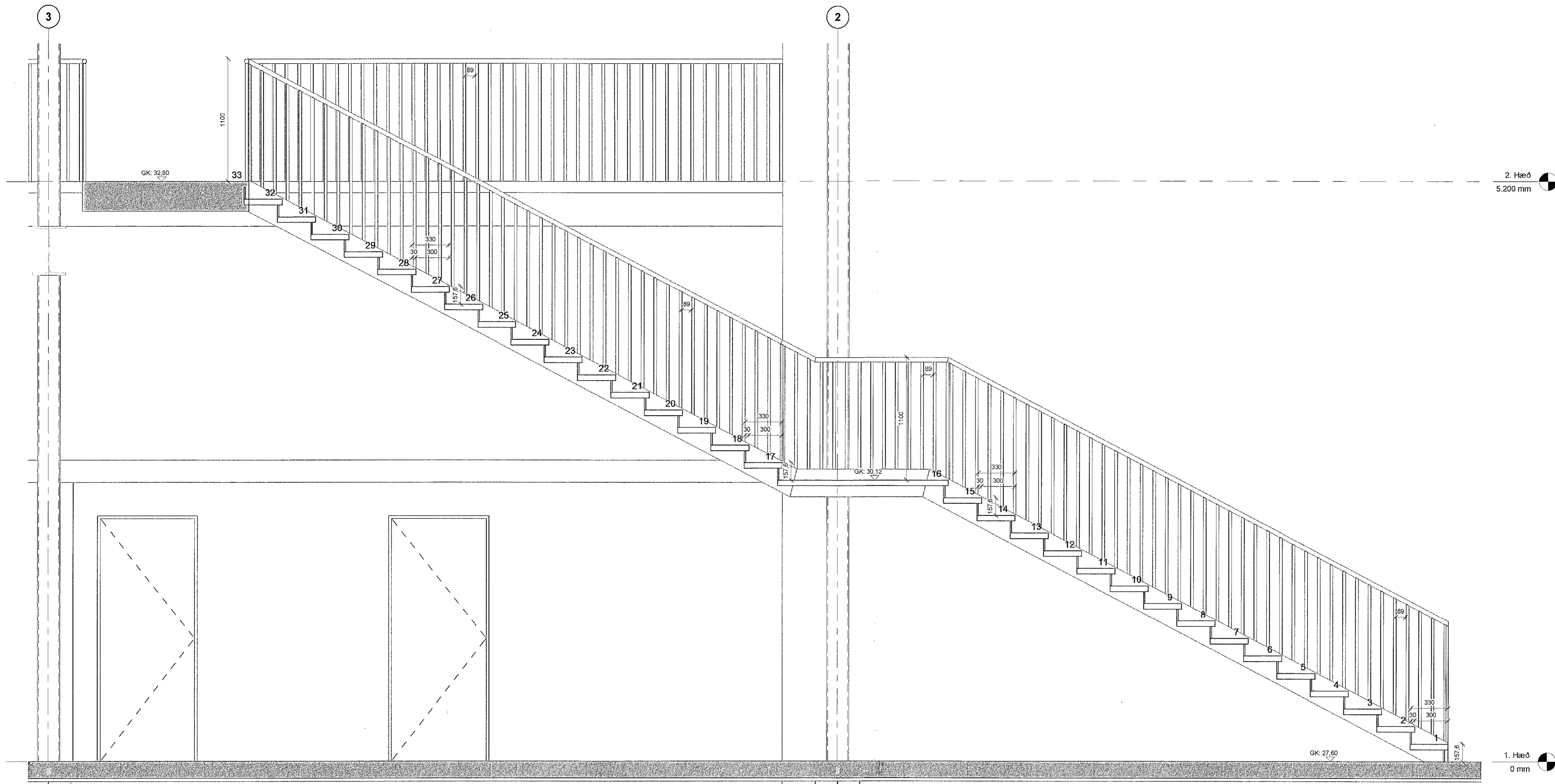
2 Stigi Framleiðslusal Snið A-A VT 1 : 20
