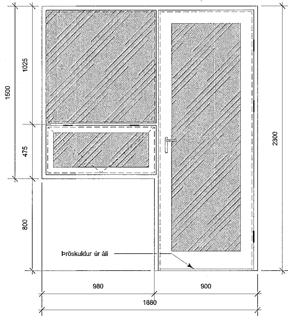
Gluggi og svalahurð. - suðurhlíð 1 stk Mkv. 1:20
