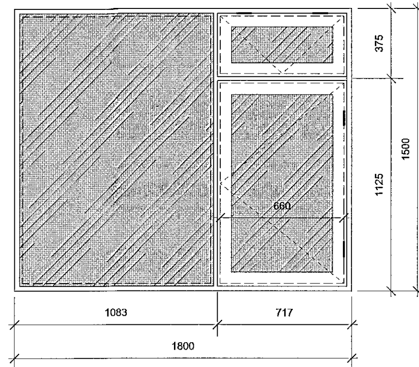
Gluggi og svalahurð. - suðurhlíð 1 stk Mkv. 1:20
