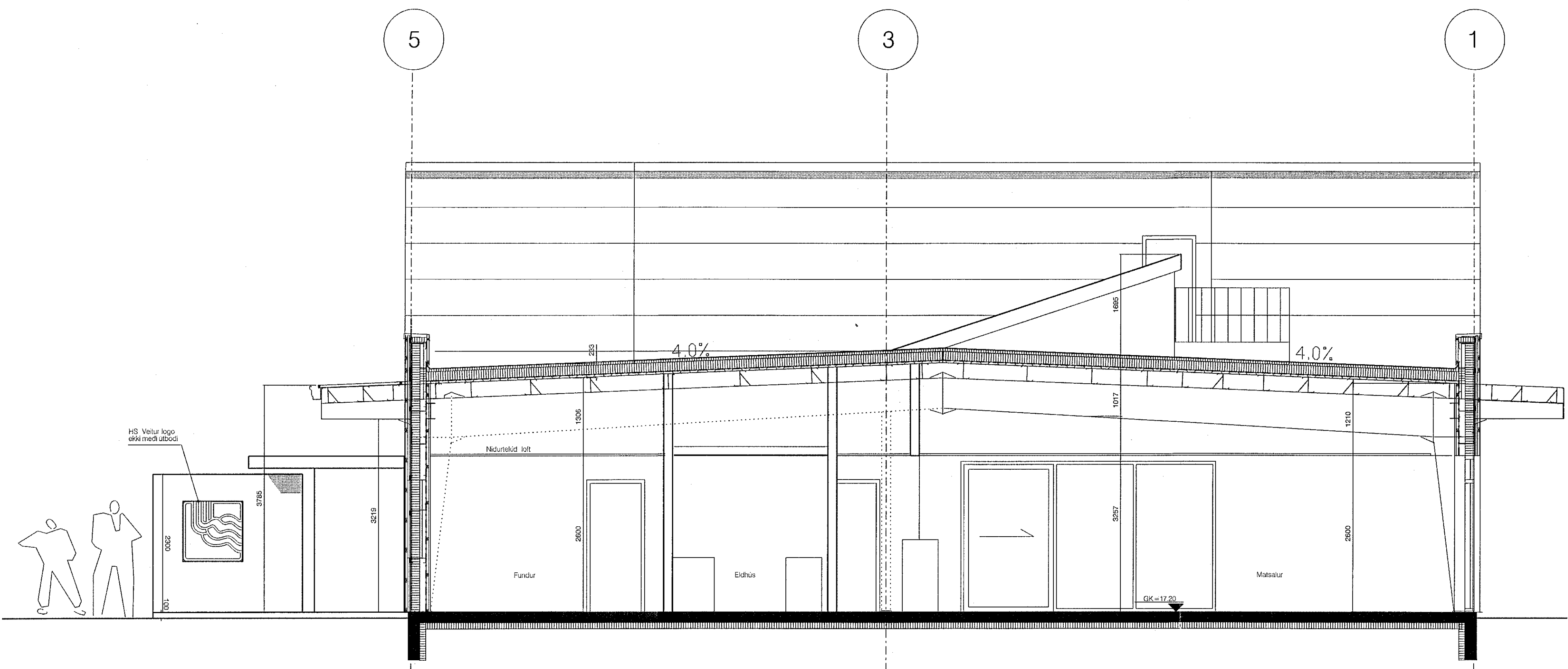
Sneid A-A
