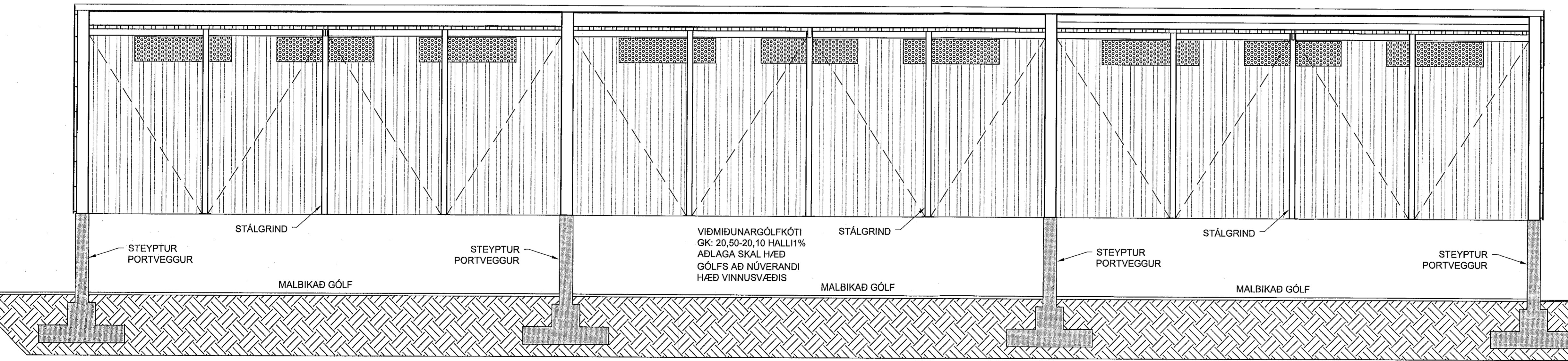
01 SNID 1:100
