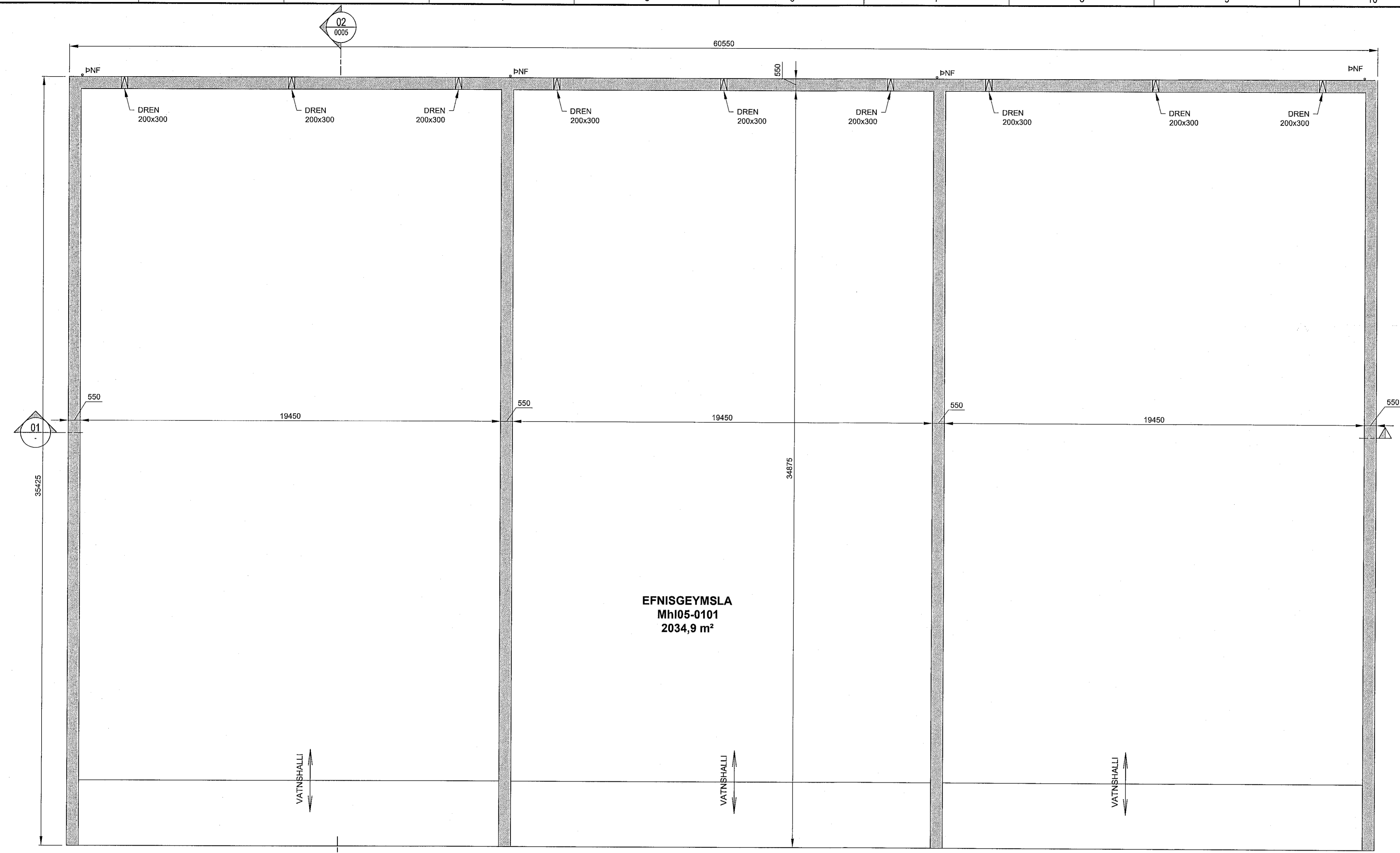
GRUNNMYND 1:100
