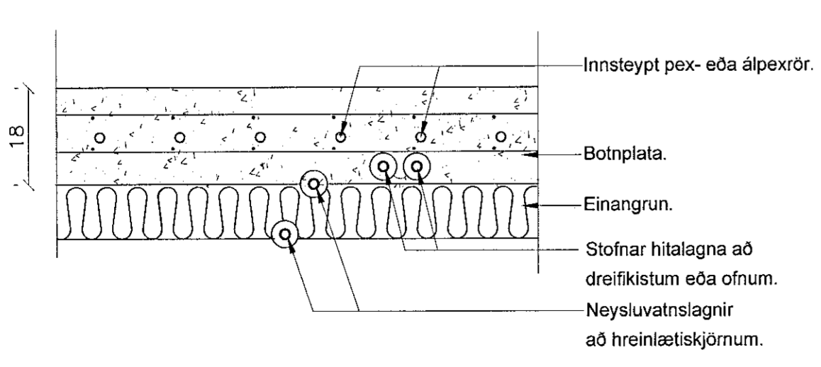
Snið í gólf verkstæði. 1:10
