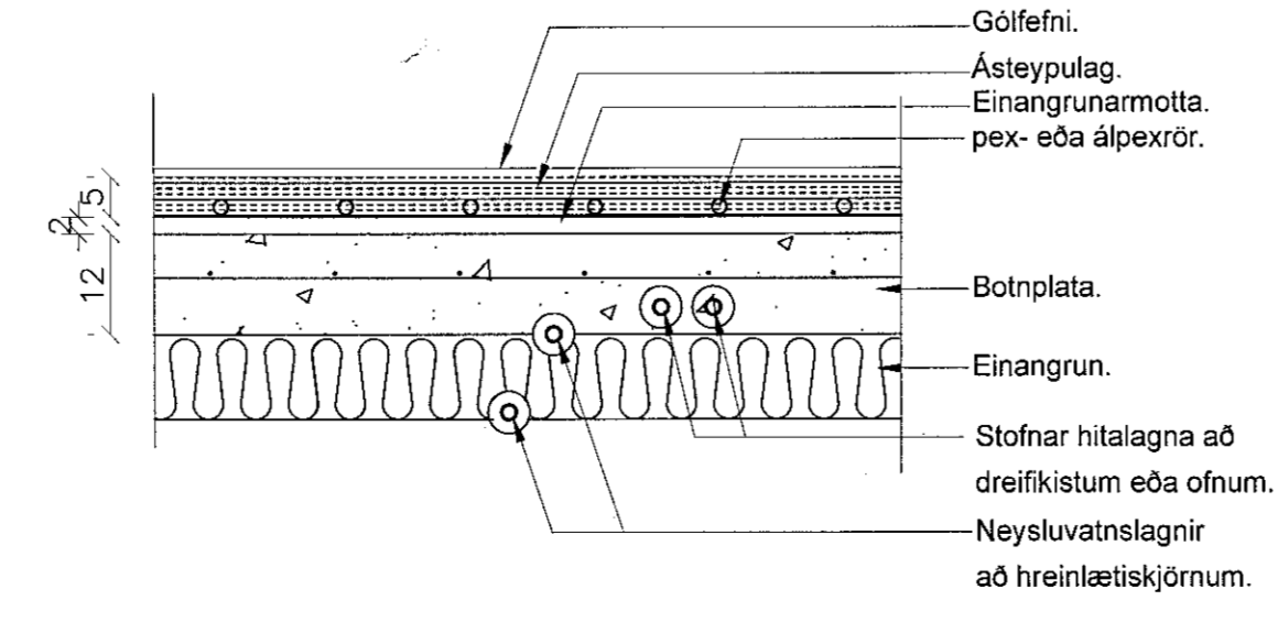
Snið í gólf skrifstofu. 1:10
