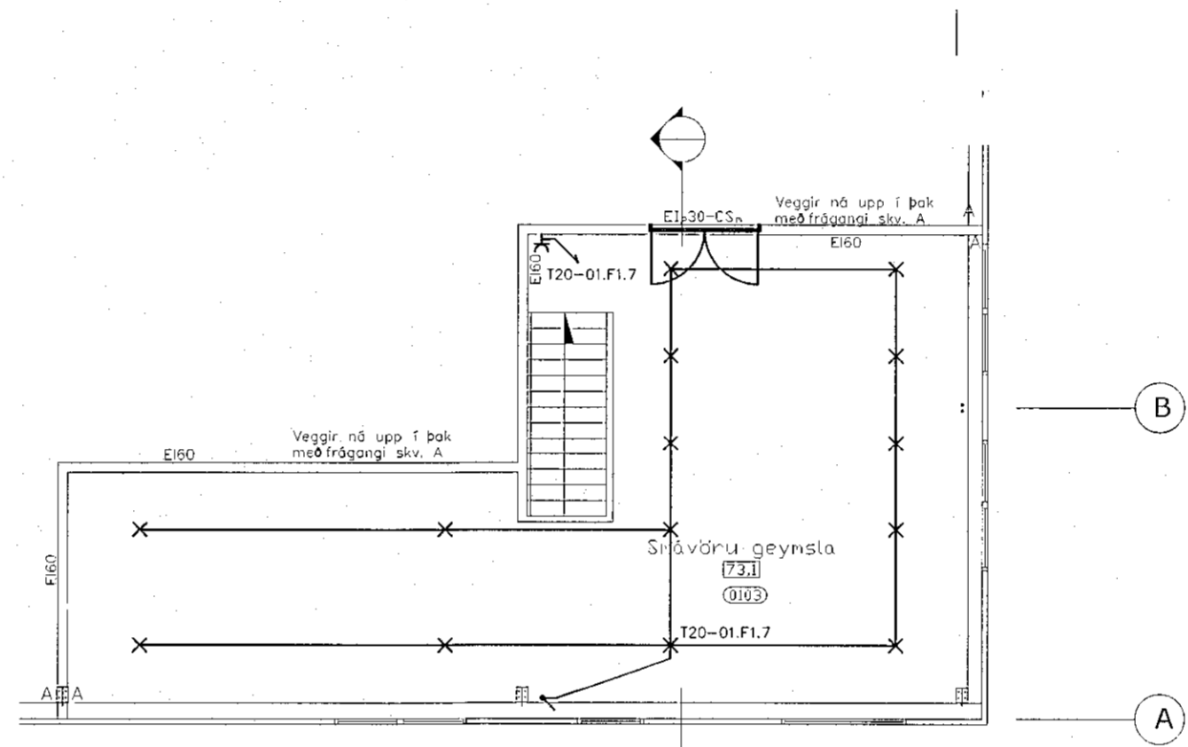
Grunnmynd 2. hæðar 1:100
