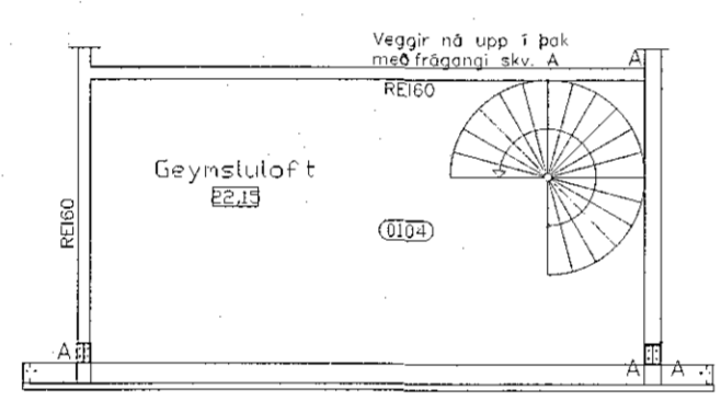
Grunnmynd 2. hæðar 1:100
