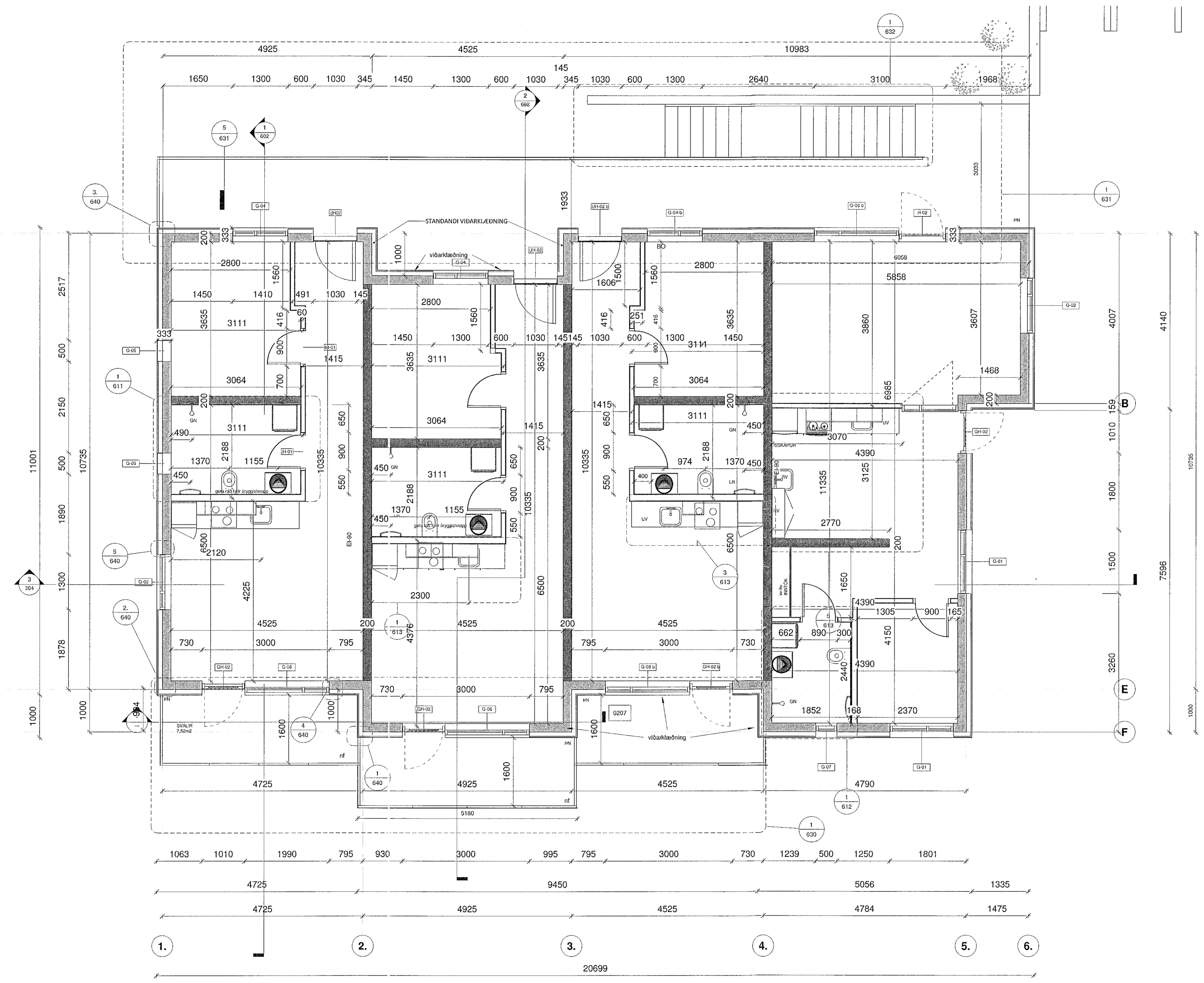
GRUNNMYND 1. HÆÐ VERKTEIKNING 1 : 50
