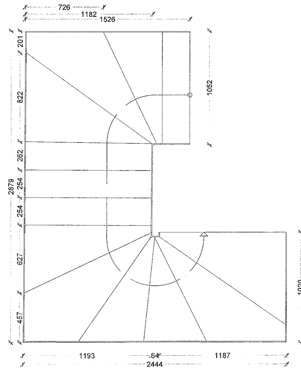
HÆÐ 2770mm STÁL-TIMBURÞREP LOKAÐ Á MILLI
