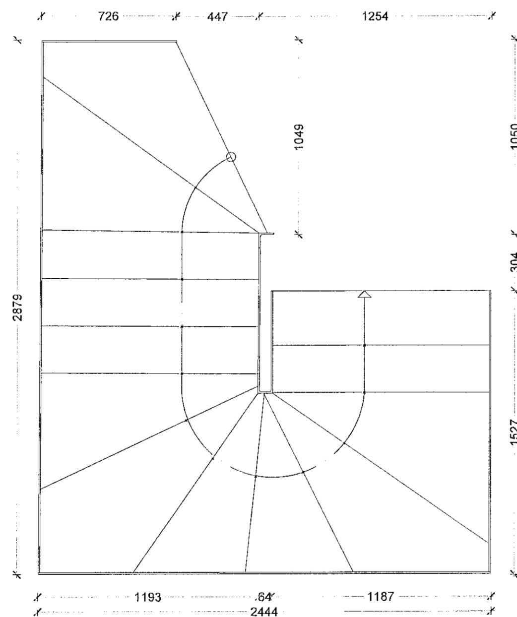
HÆÐ 2770mm STÁL-TIMBURÞREP OPID Á MILLI
