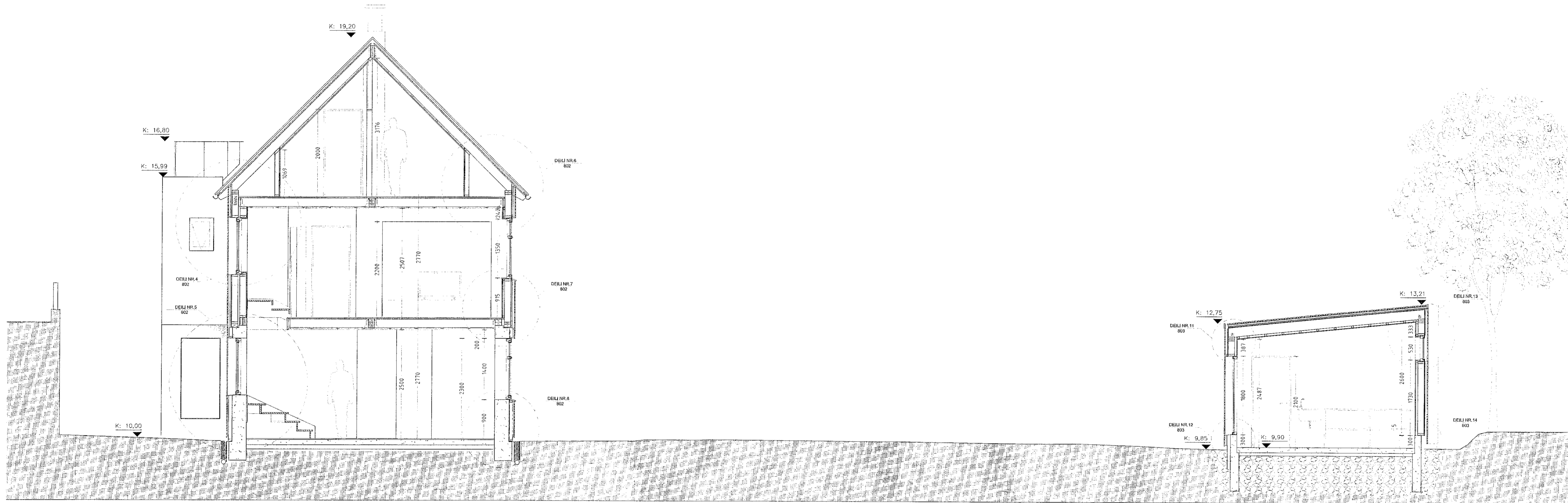
SNID A-A MKV 1:50
