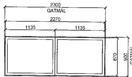
G-03 1 STK SAMTALS ÁLTIMBURGLUGGI LITIR VELJIST Í SAMRÁÐI VIÐ ARKITEKT
