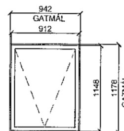
G-04 2 STK SAMTALS ÞAKGLUGGI, RAFSTYRÐ OPNUN LITIR VELJIST Í SAMRÁÐI VIÐ ARKITEKT
