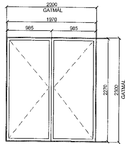
UH-01 1 STK SAMTALS ÁLTIMBURHURÐ LITIR VELJIST Í SAMRÁÐI VIÐ ARKITEKT
