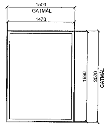
G-01 2 STK SAMTALS ÁLTIMBURGLUGGI LITIR VELJIST Í SAMRÁÐI VIÐ ARKITEKT
