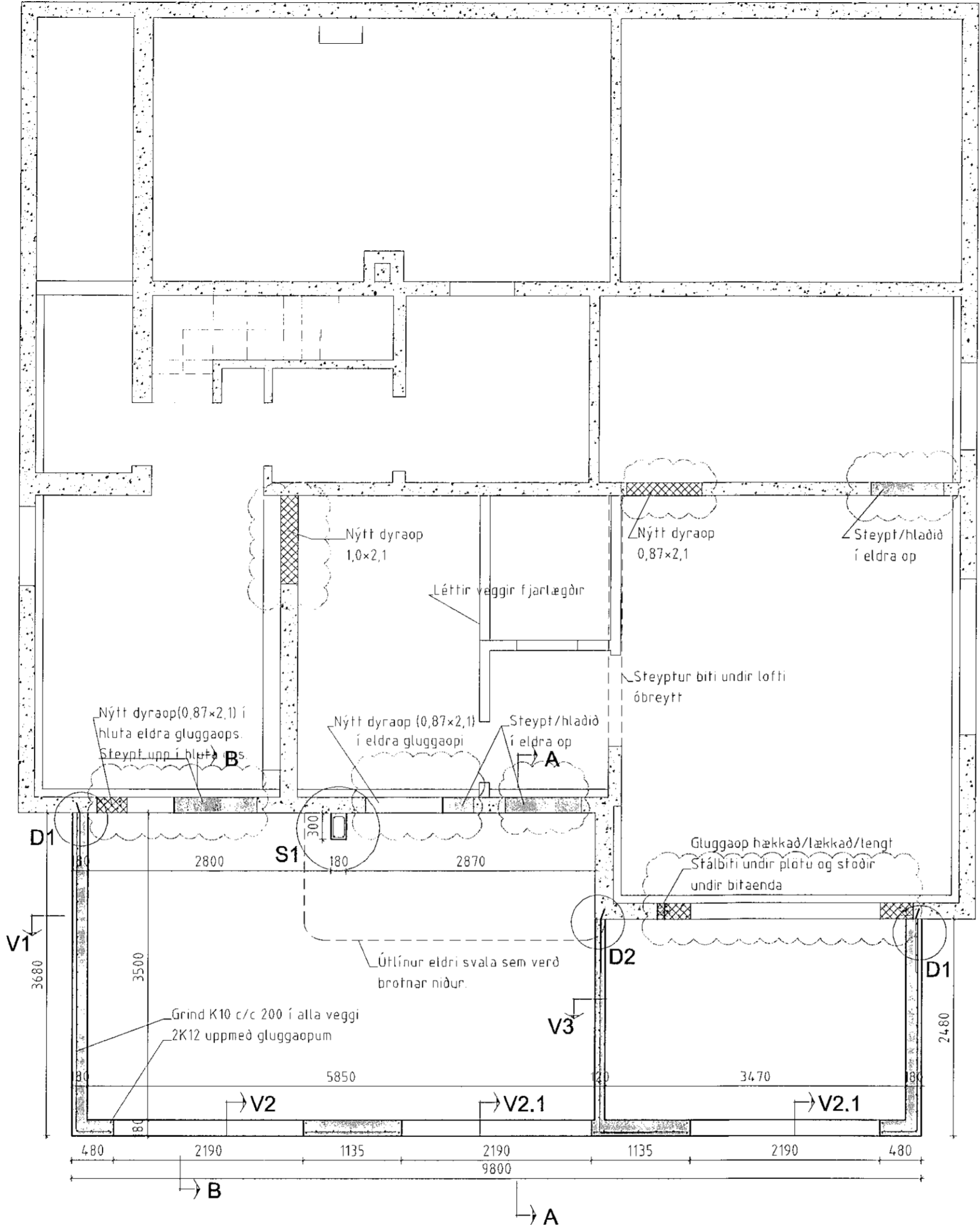
Jarðhæð - Grundmynd - 1:50
