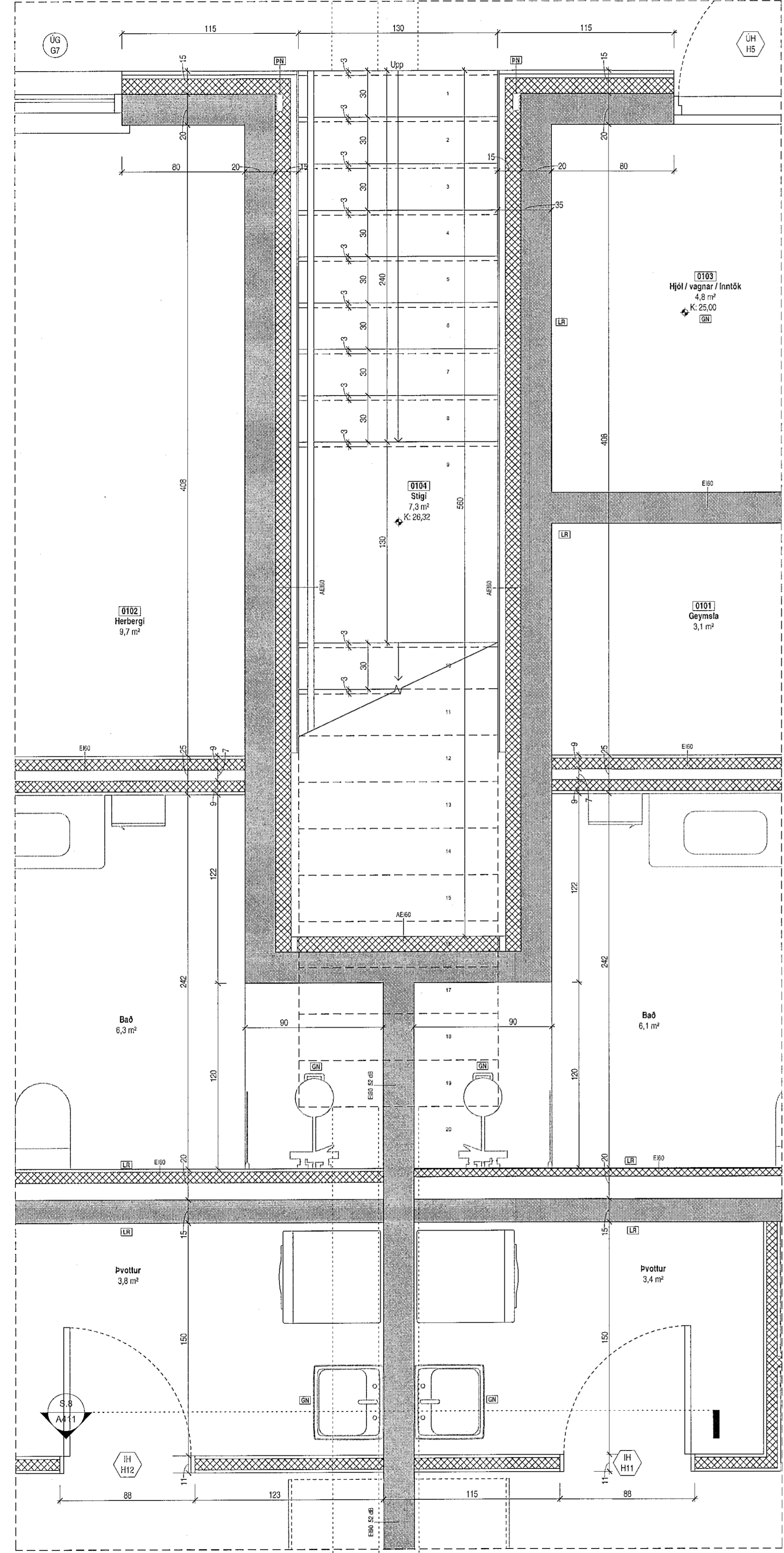
Stigateikning grunnmynd 1.hæð 1:20
