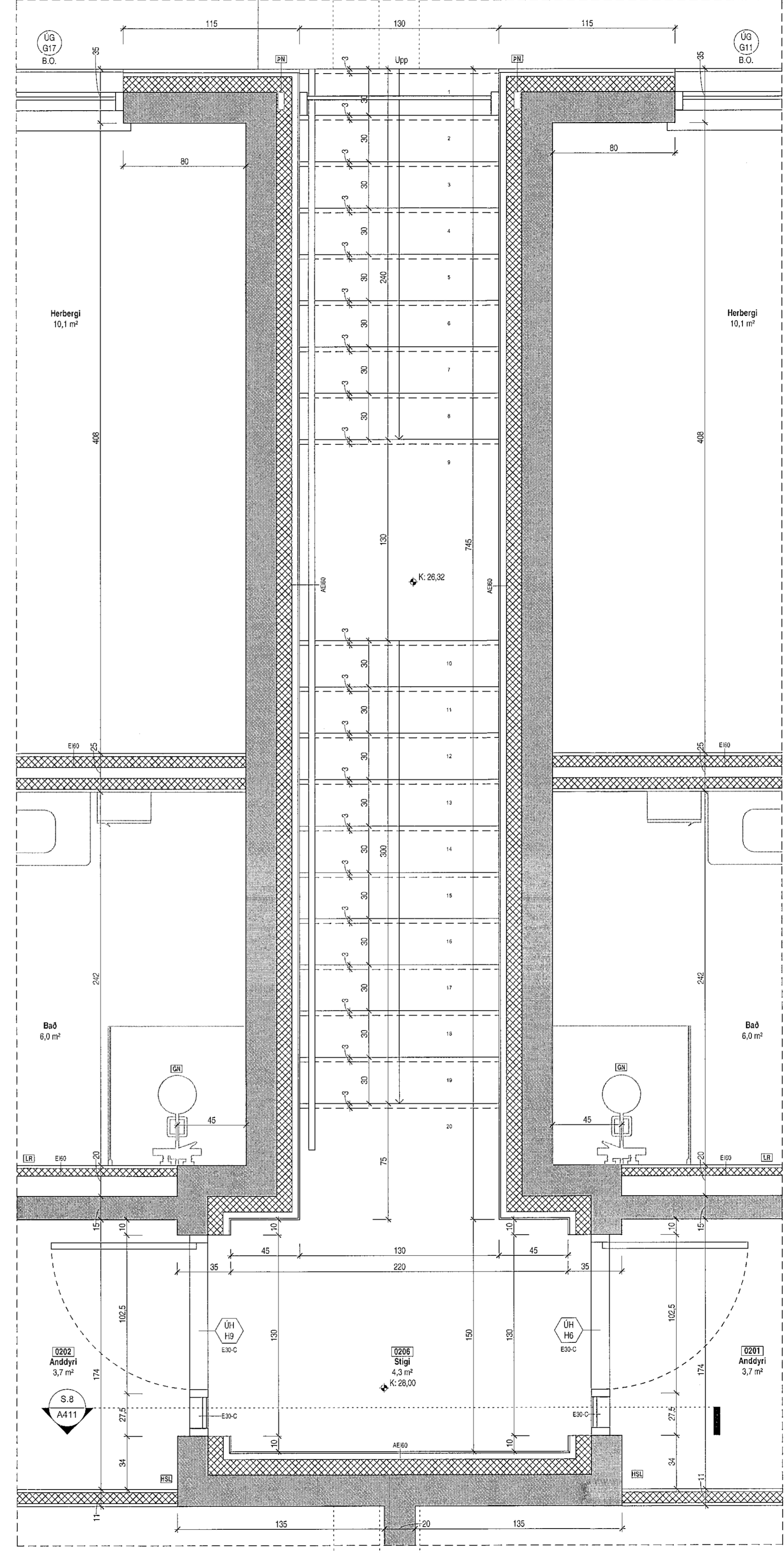
Stigateikning grunnmynd 2.hæð 1:20
