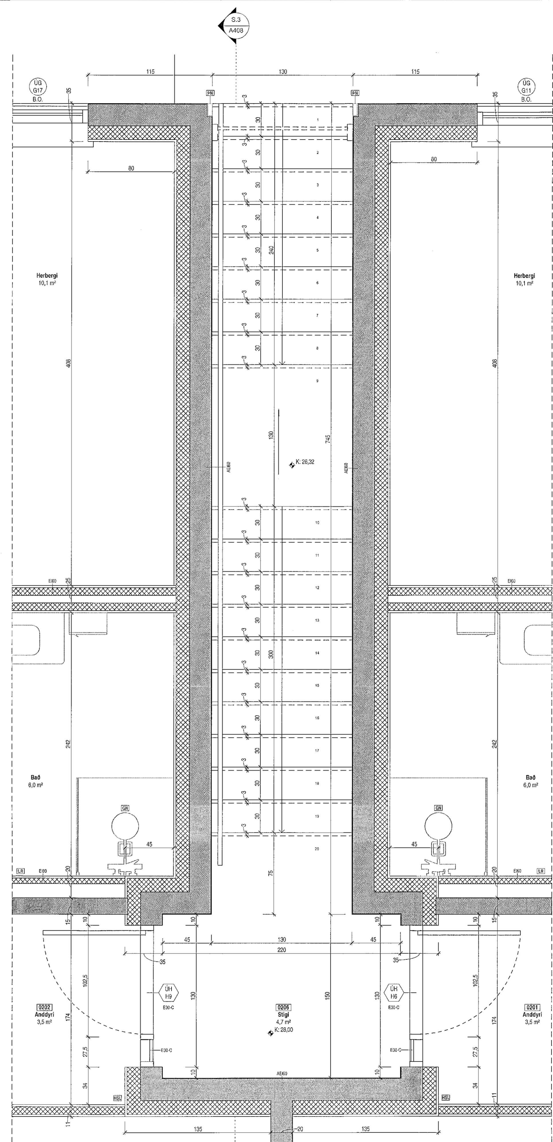
Stigateikning grunnmynd 2.hæð 1:20
