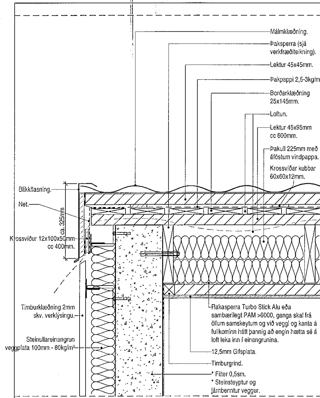
Deili 16 Nr.1 - A403 1 : 10
