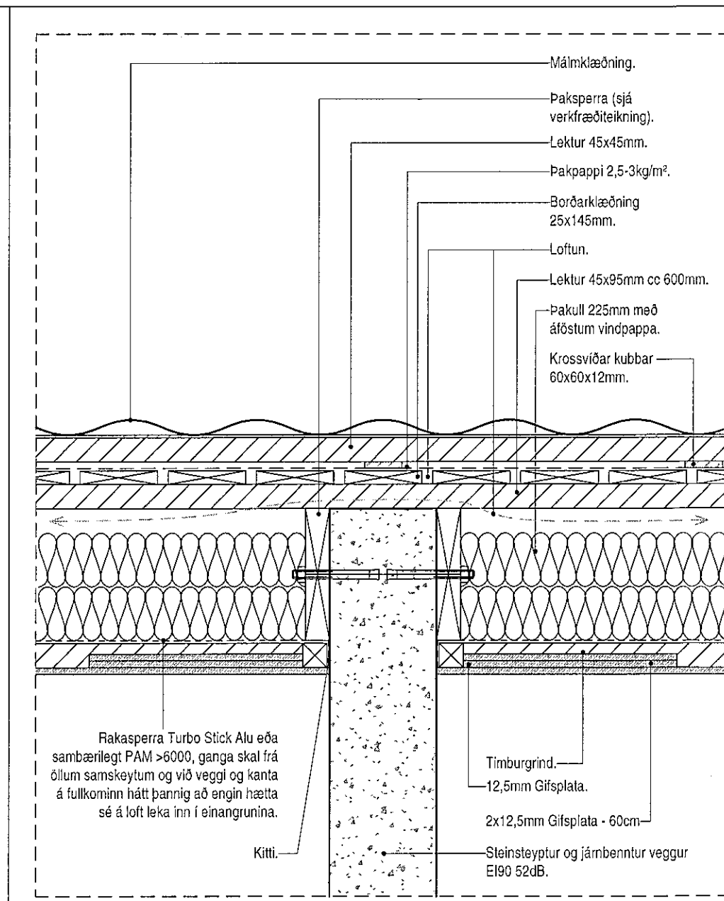
Deili 17 Nr.1 - A402 1 : 10
