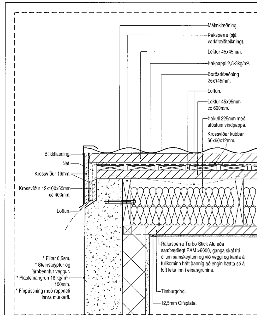
Deili 16 Nr.3-7 - A403 1 : 10
