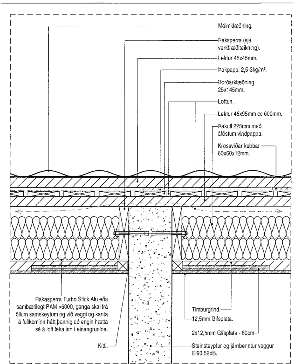
Deili 17 Nr.3-7 - A407 1 : 10
