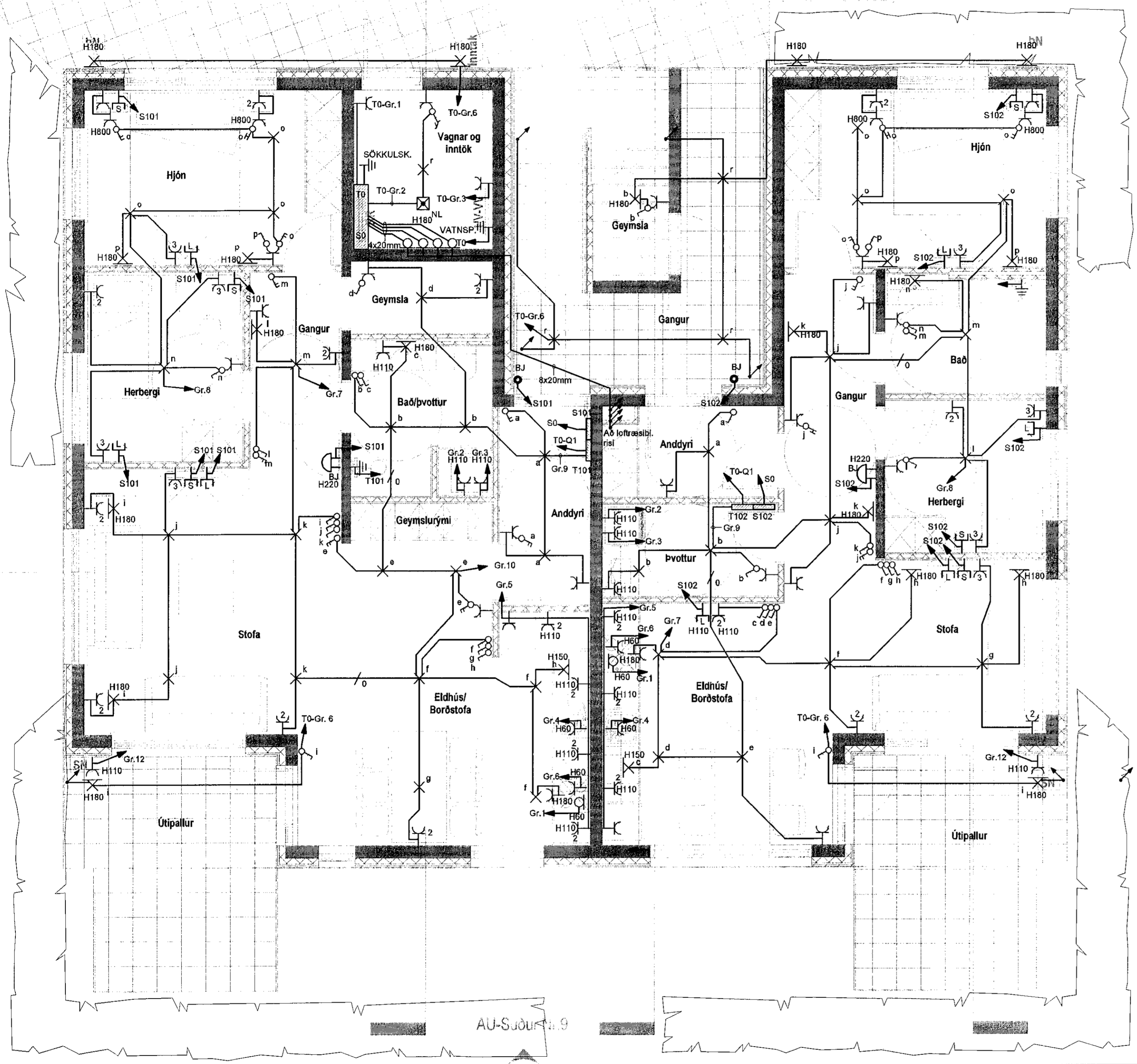
GRUNNMYND 1.HÆÐ Mkv. 1:50
