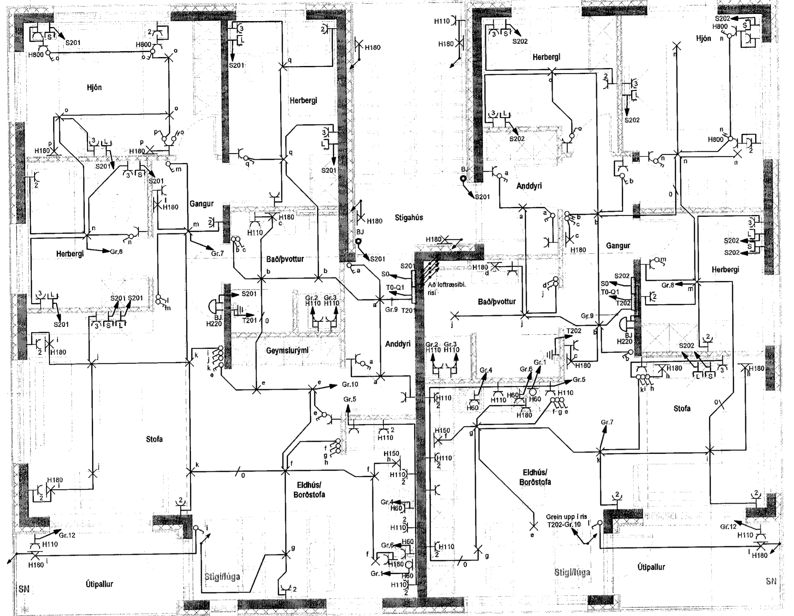
GRUNNMYND 2.HÆÐ Mkv. 1:50
