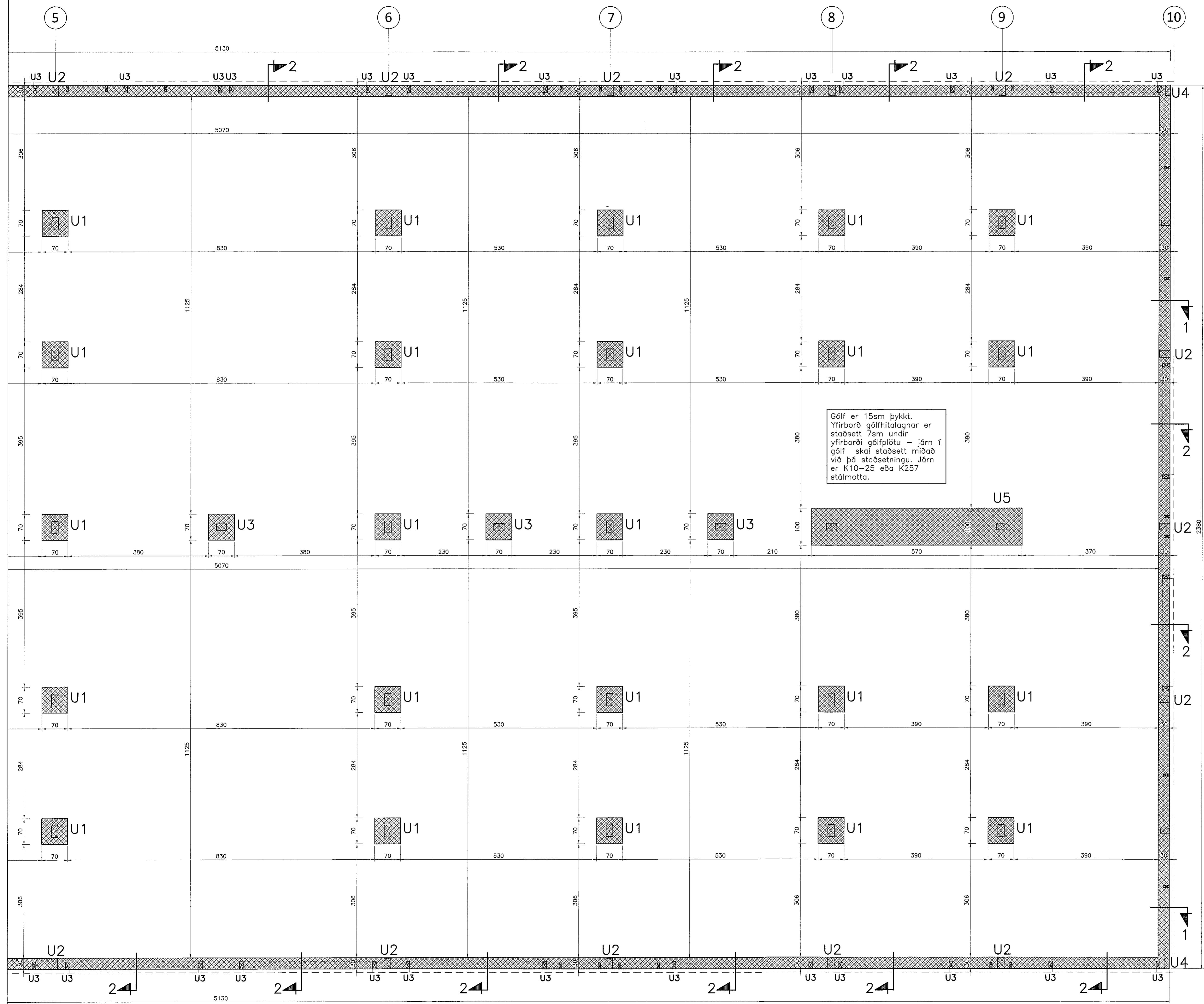
Grunnmynd undirstaða (milli lína 5-10) 1:50
