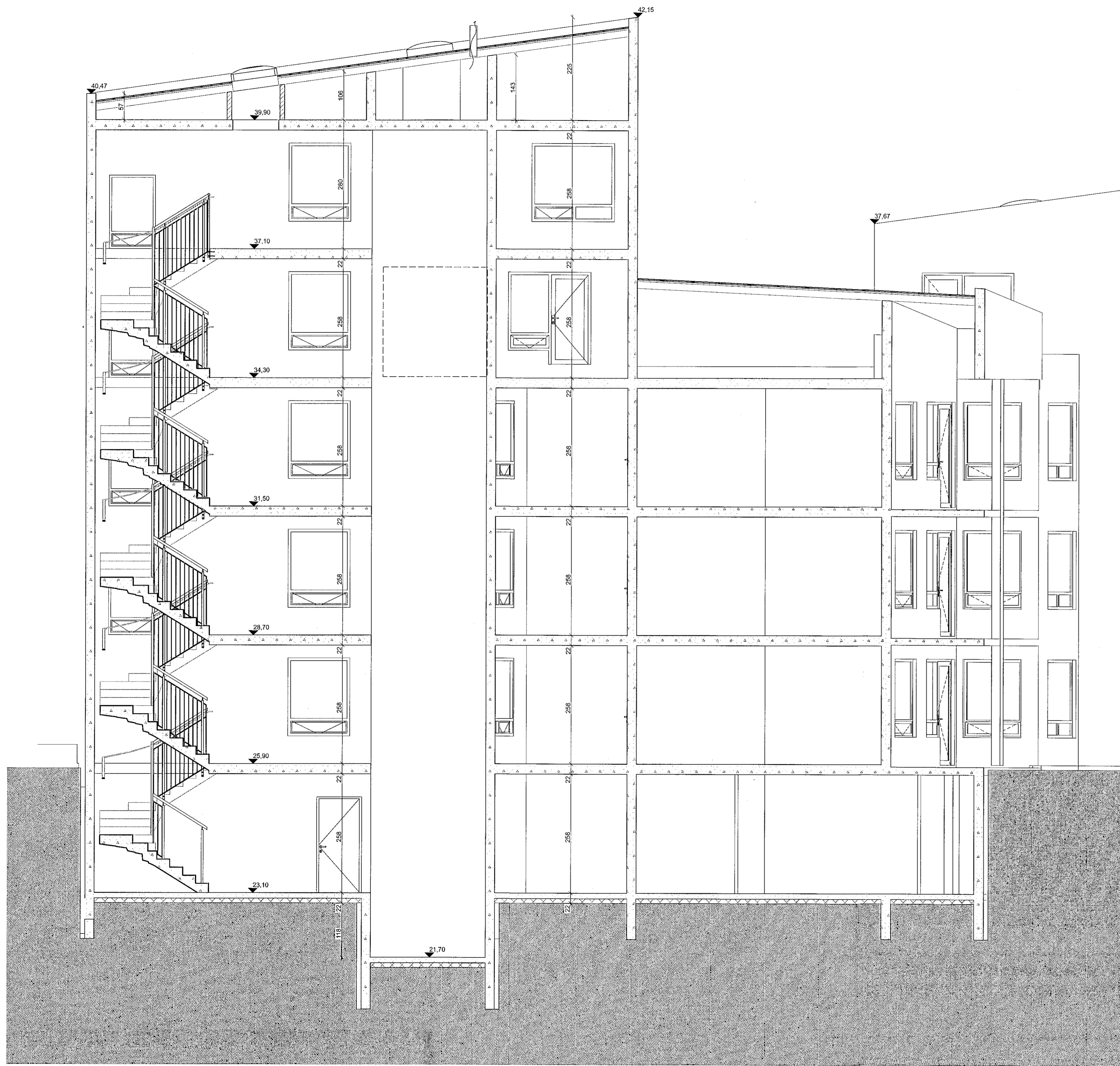
B-B
