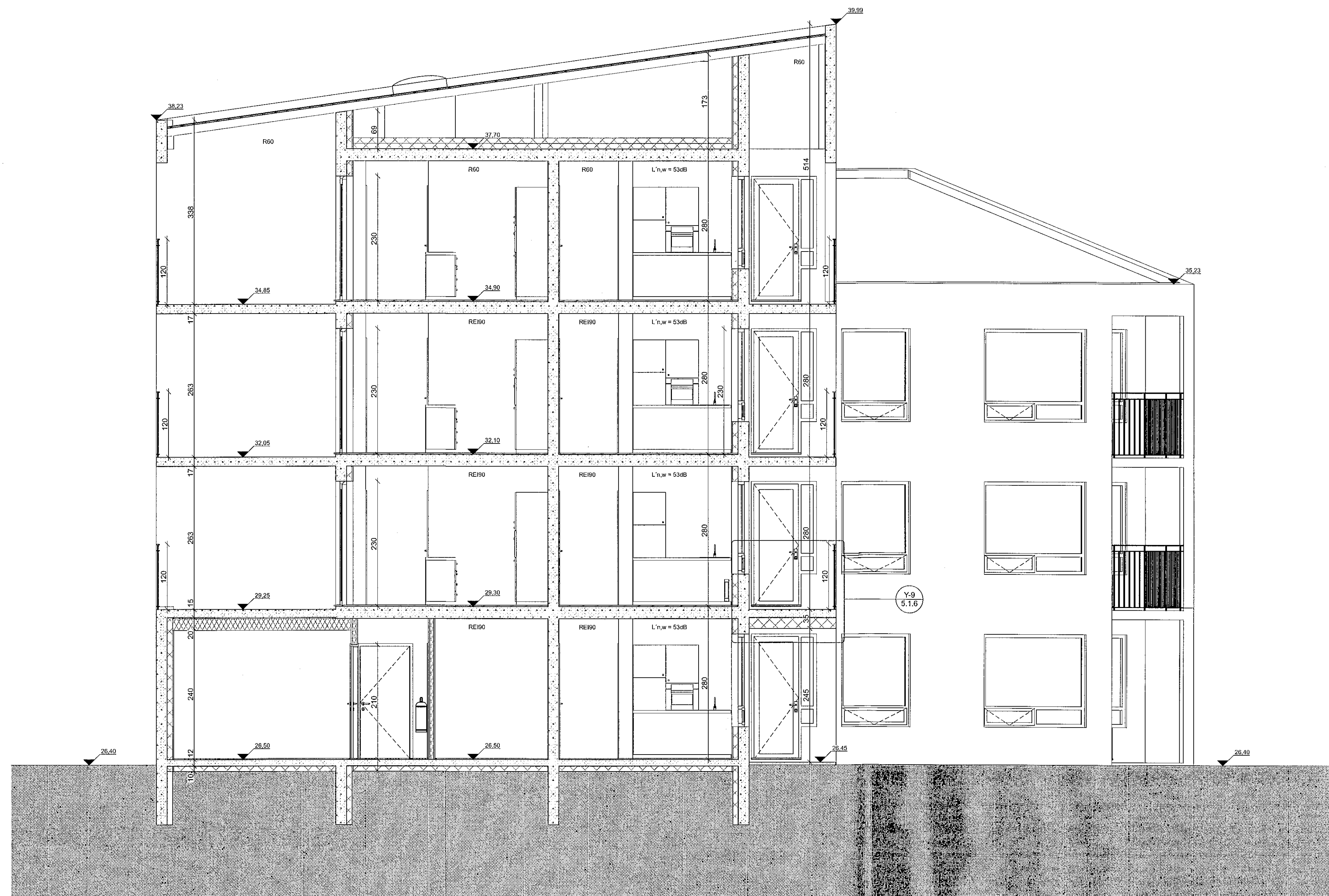
A-A snið
