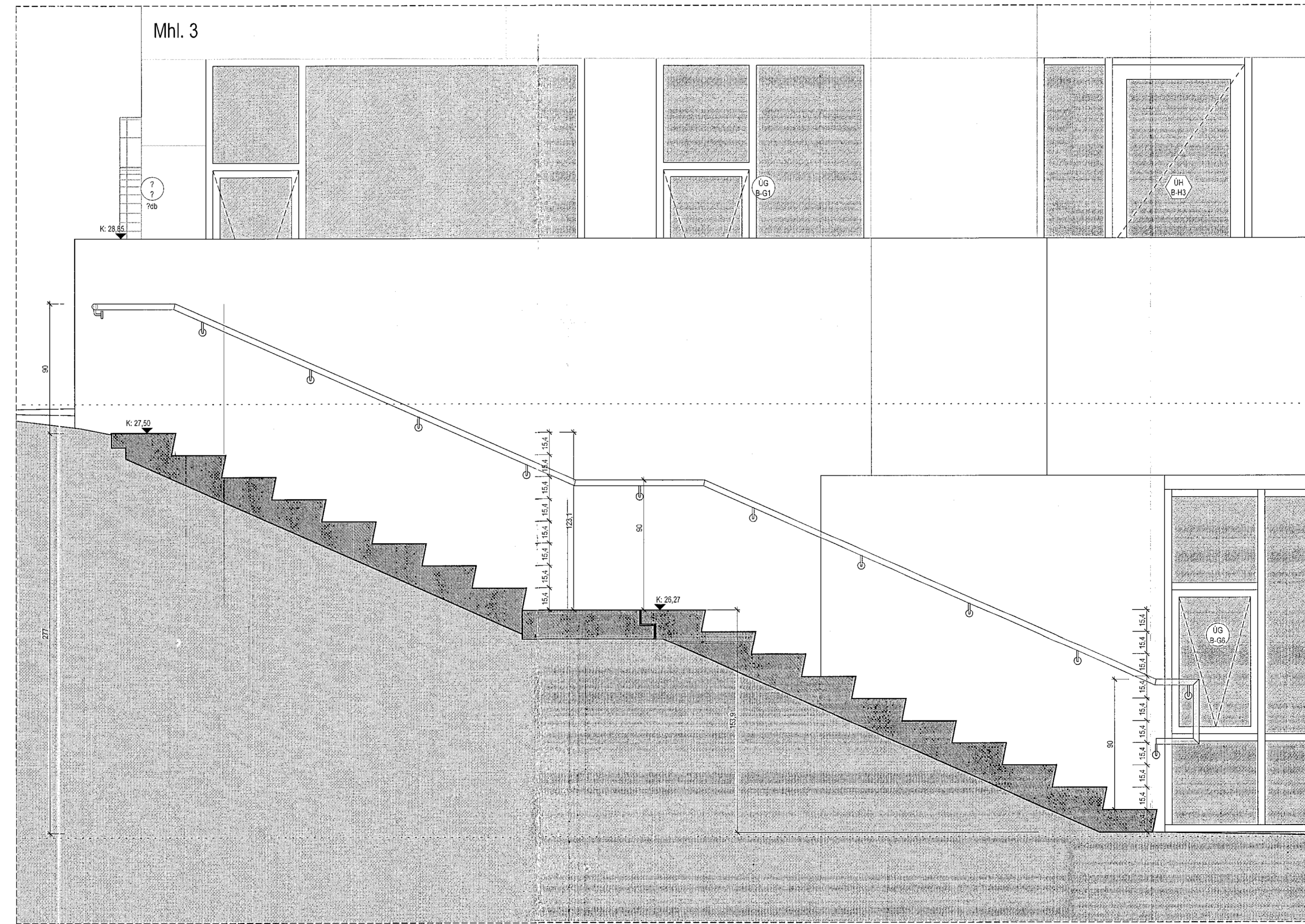
Úttröppur. Sníð 1:20
