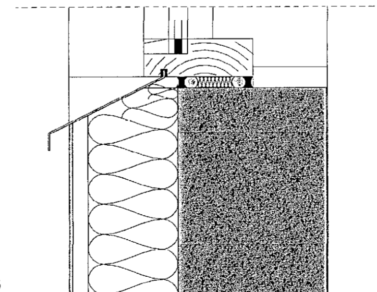
Glugga deilir neðripartur 1 : 5
