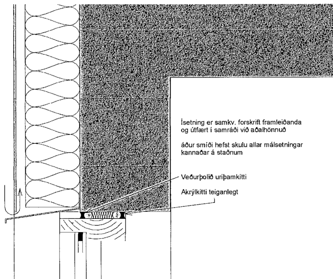
Glugga deilir efripartur 1 : 5
