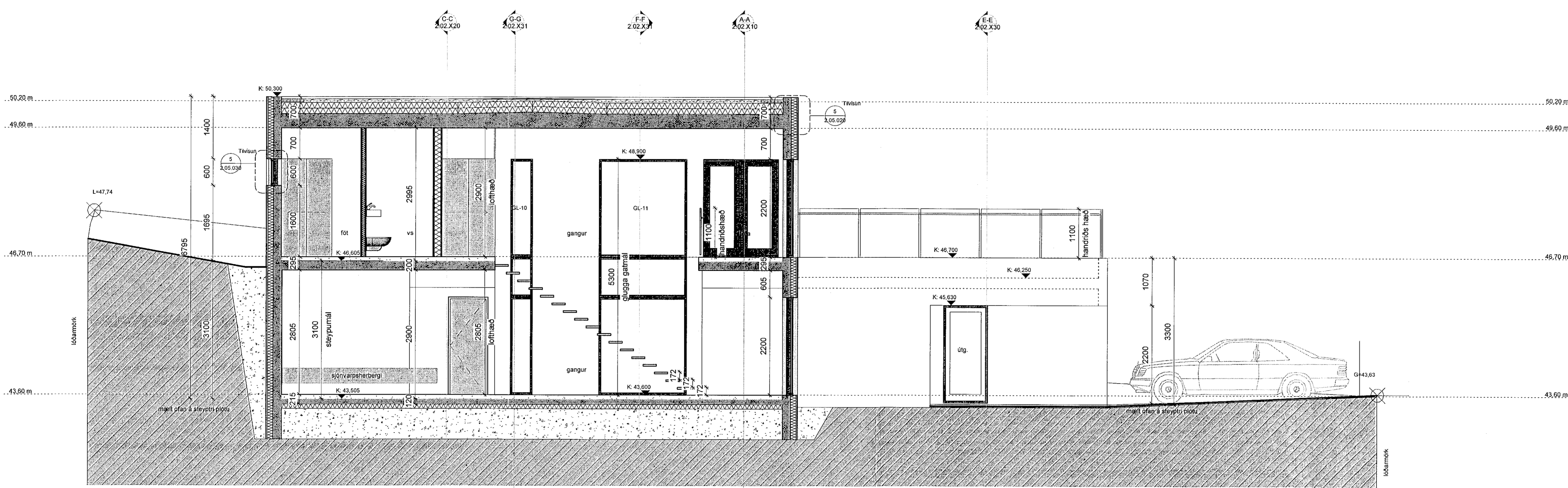
A-A 1.0-SNEIÐING A-A 1:50
