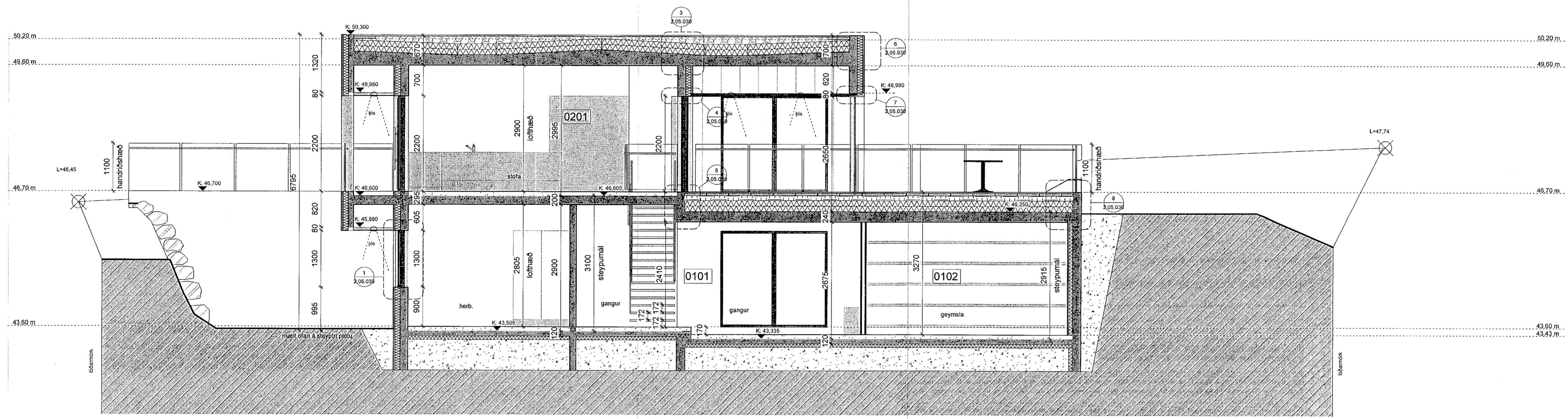
A-A 1.0-SNEIÐING A-A 1:50
