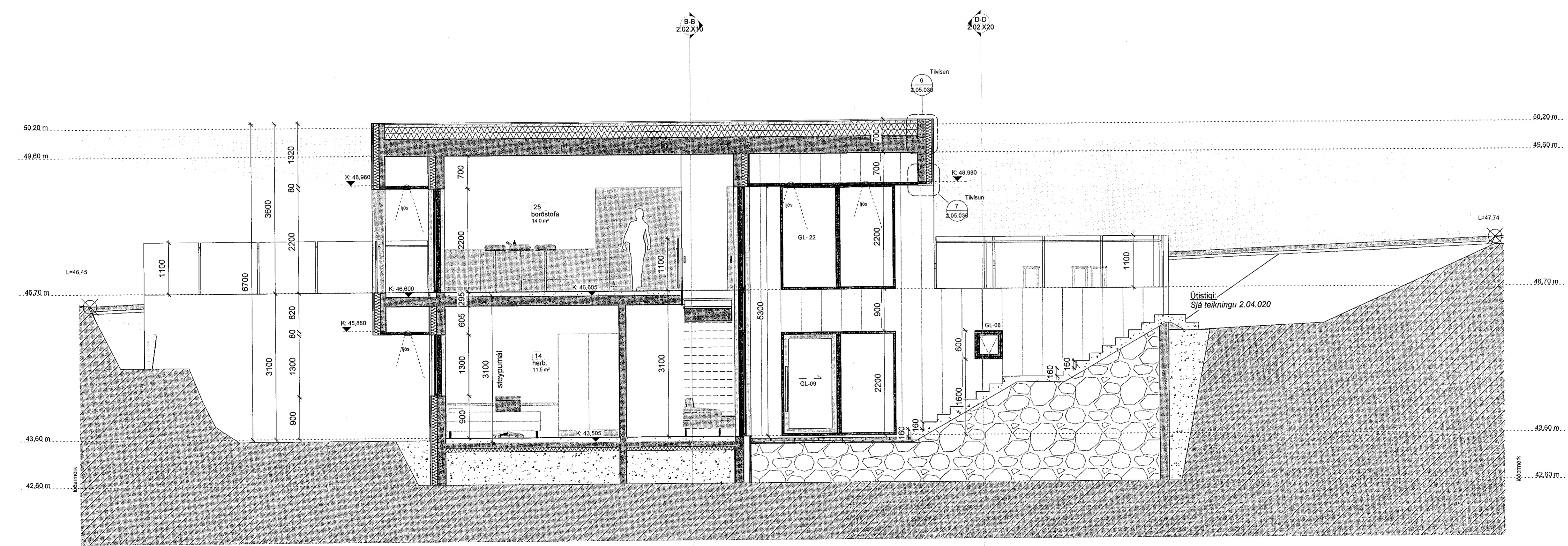
7.0-SNEIDING G-G 1:50
