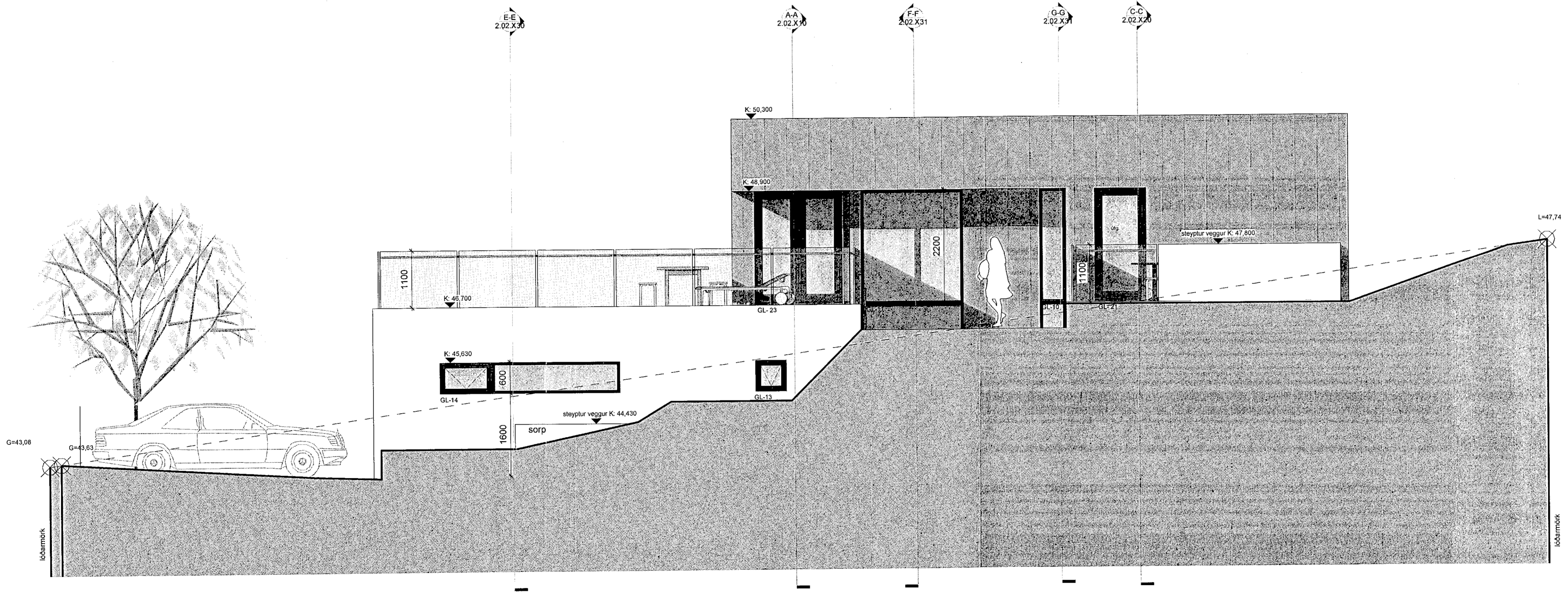
ÚTLIT - AUSTUR 1:50
