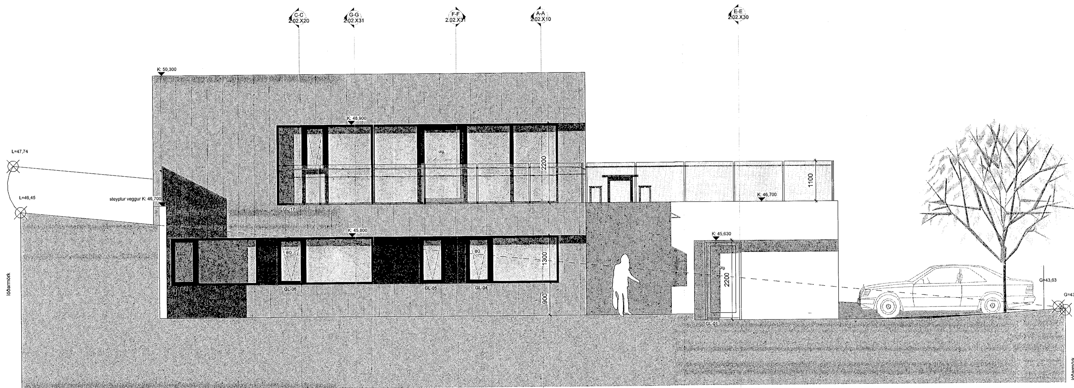
ÚTLIT - VESTUR 1:50
