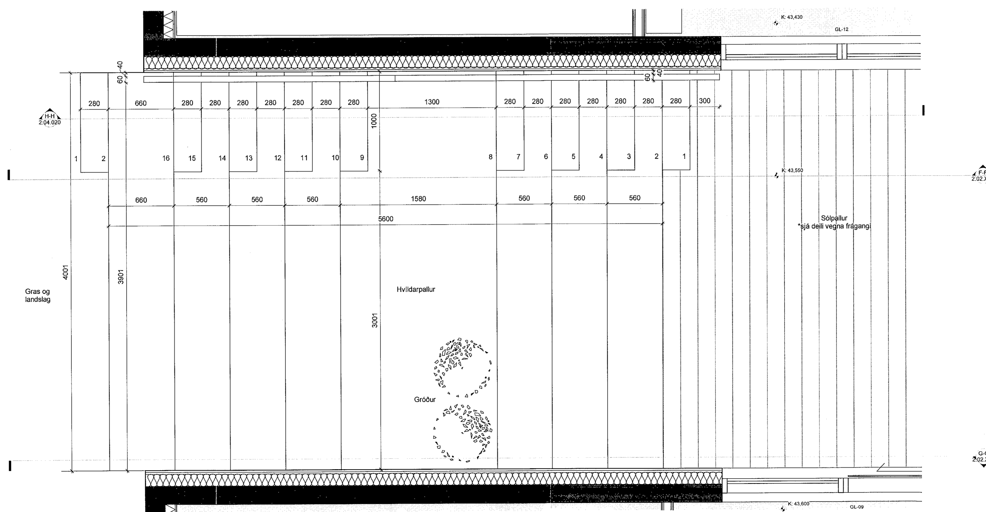
1.0-GRUNNMYND - Útistíga 1:20
