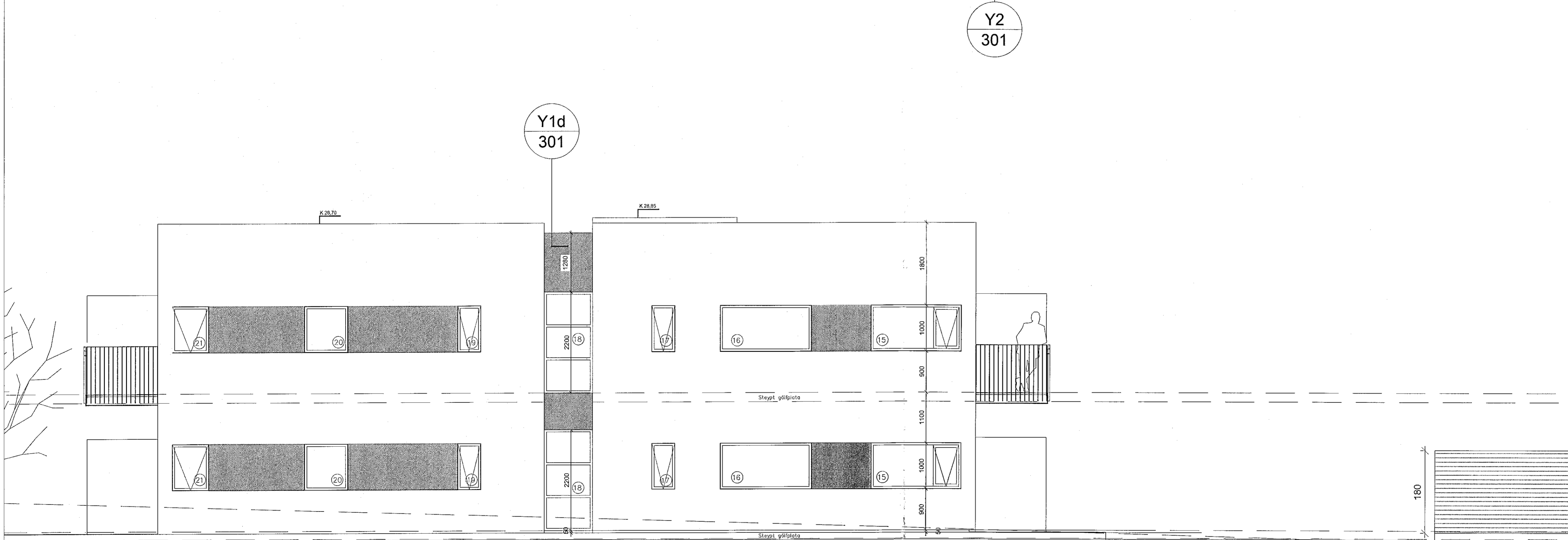
Norðurhella 1:50
