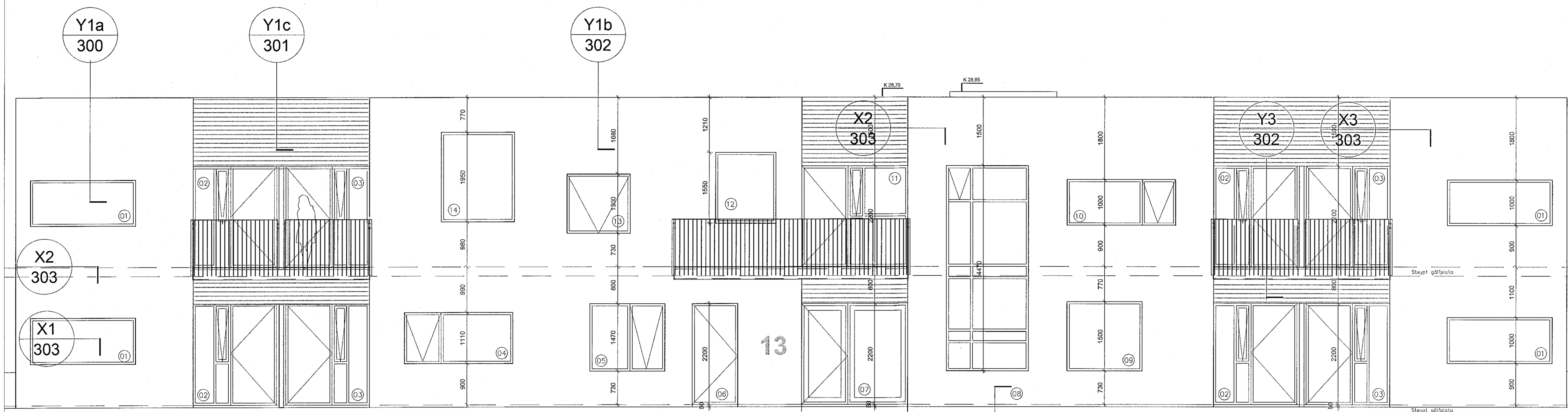
Vesturhlíð 1:50
