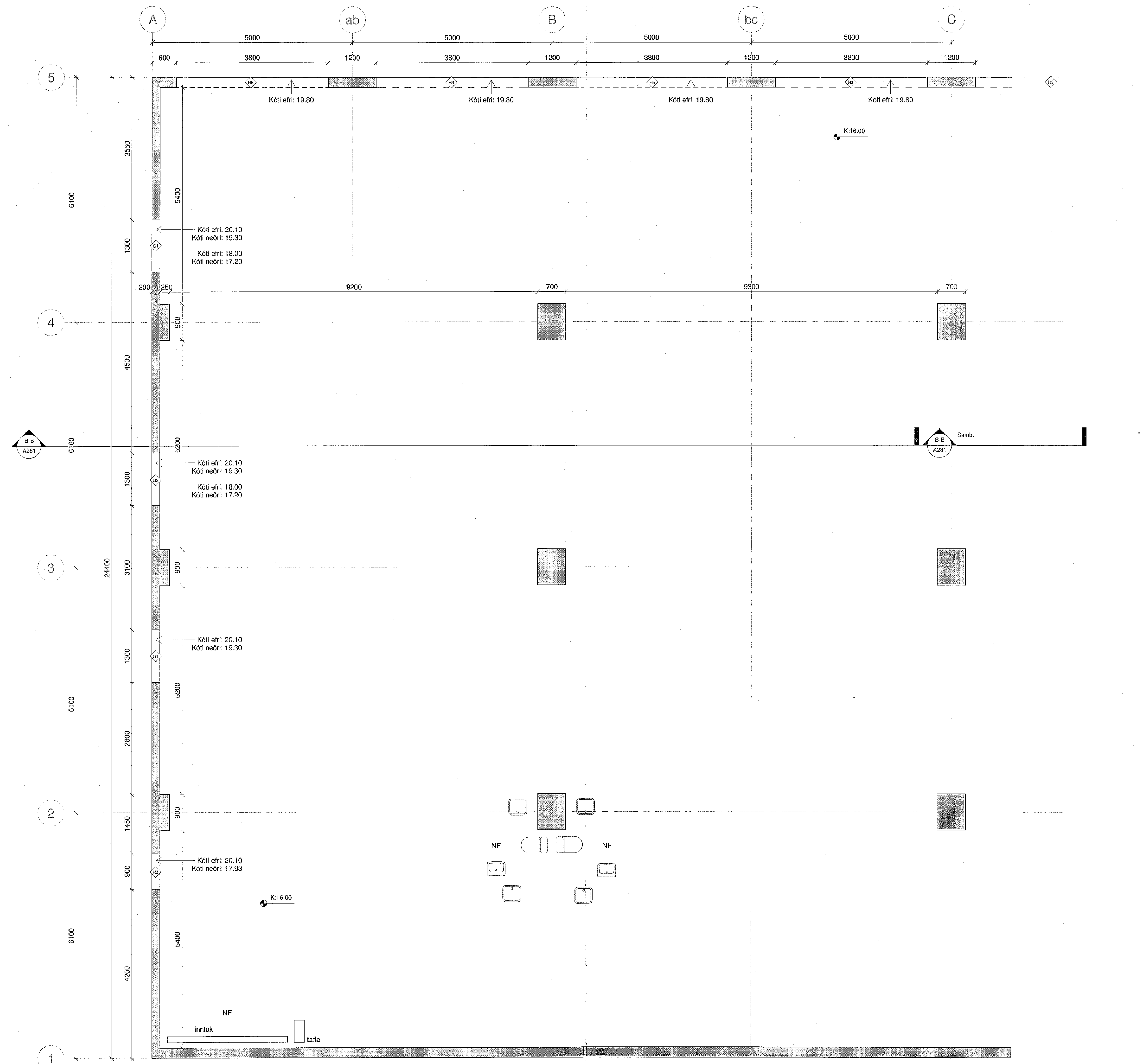
STEYPU TEIKNING 1. HÆÐ 1 : 50
