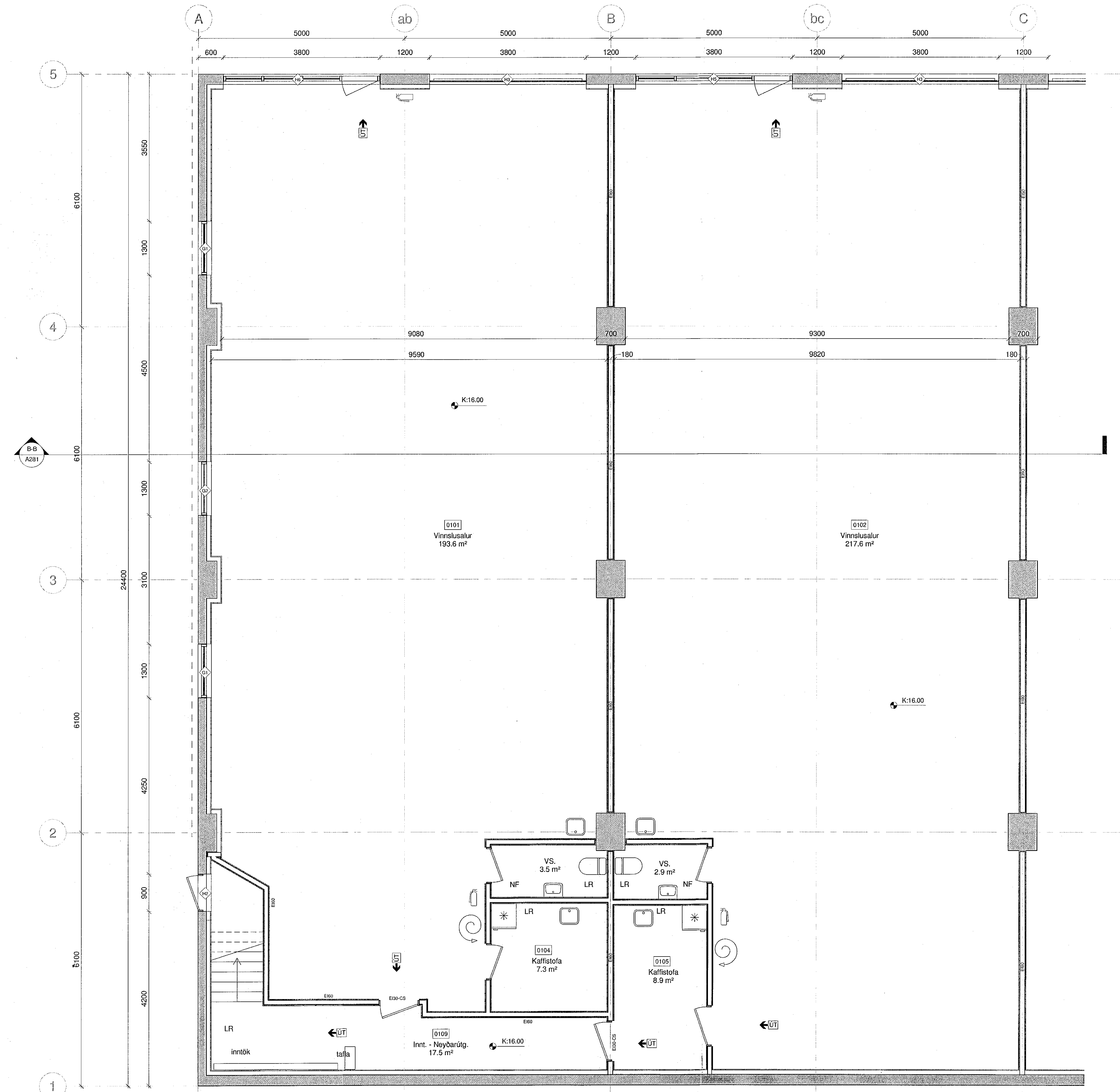
FRÁGANGUR 1. HÆÐ 1 : 50
