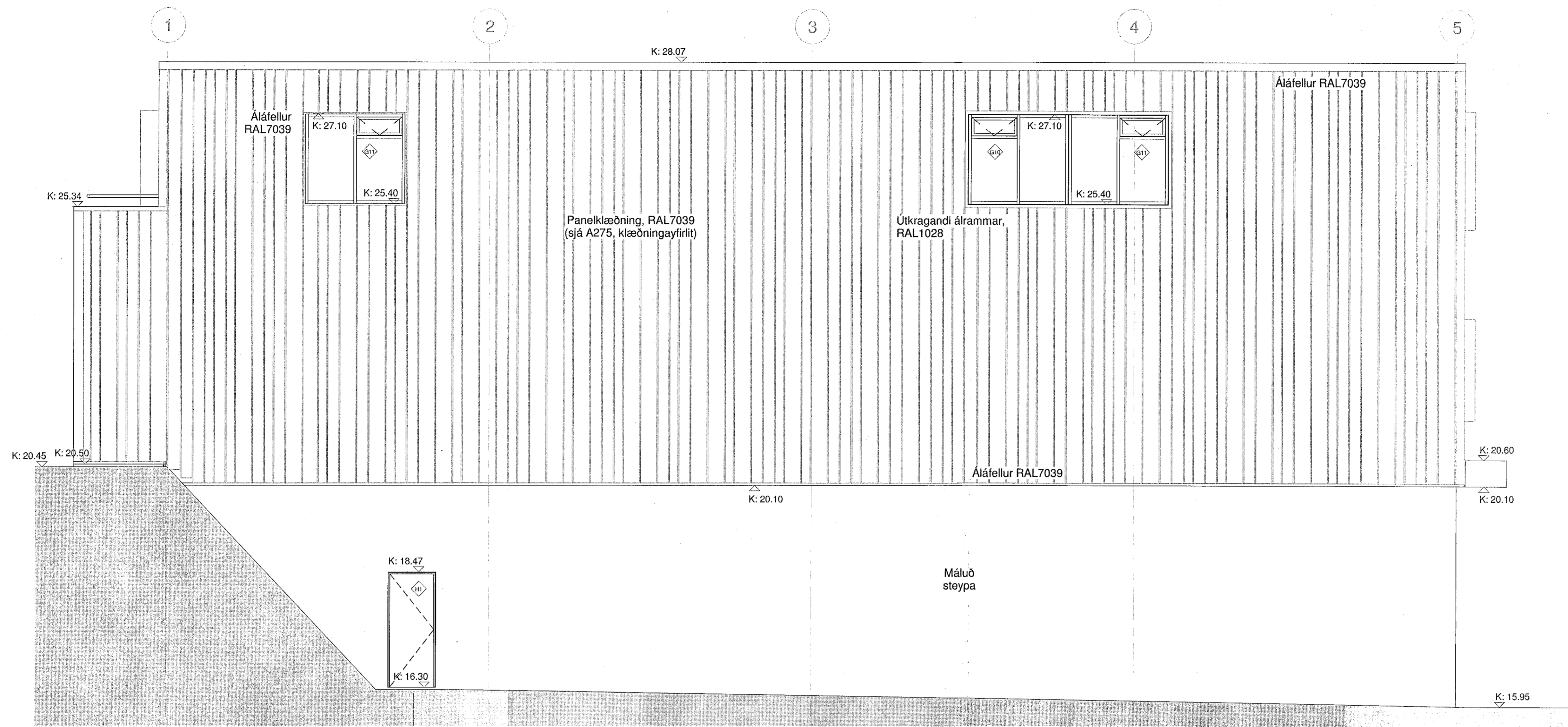
AUSTUR 1 : 50
