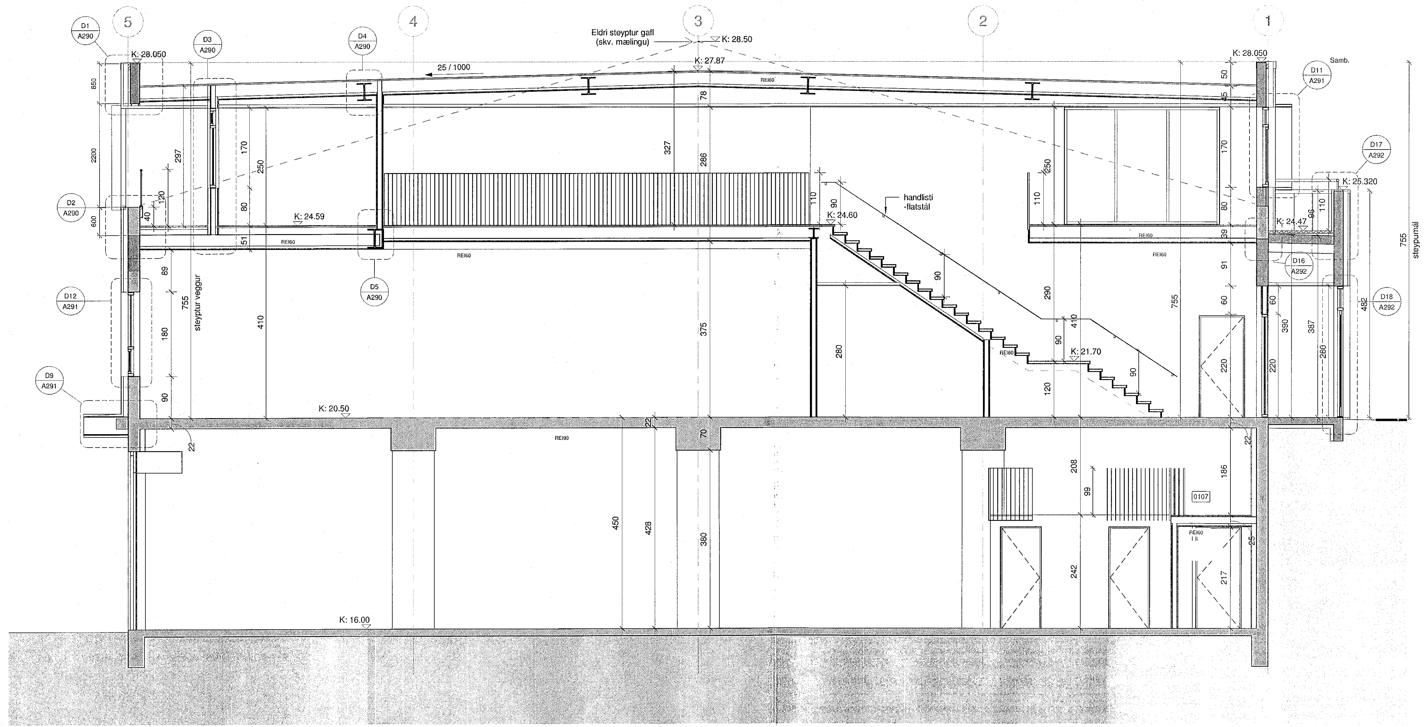
SNEIÐING A-A 1 : 50
