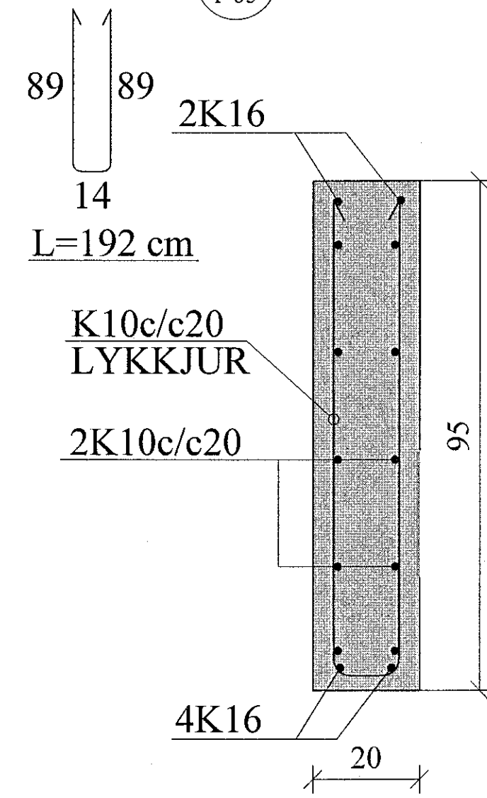
B5 SNID. 1:10
