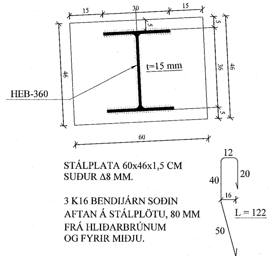
SM1 SÉRMYND. 1:10 1-11
