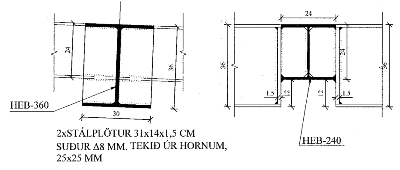
SM3 SÉRMYND. 1:10 1-11
