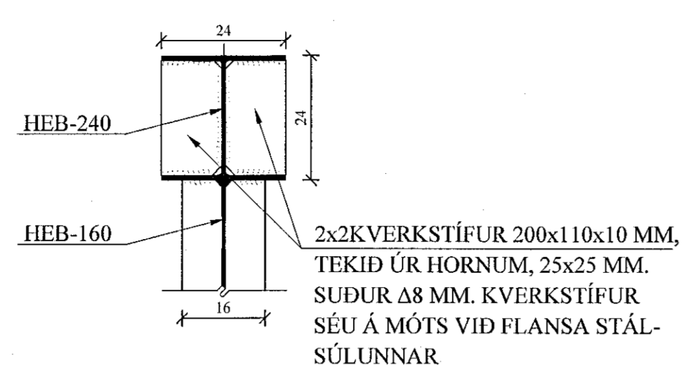
SM2 SÉRMYND. 1:10 1-11
