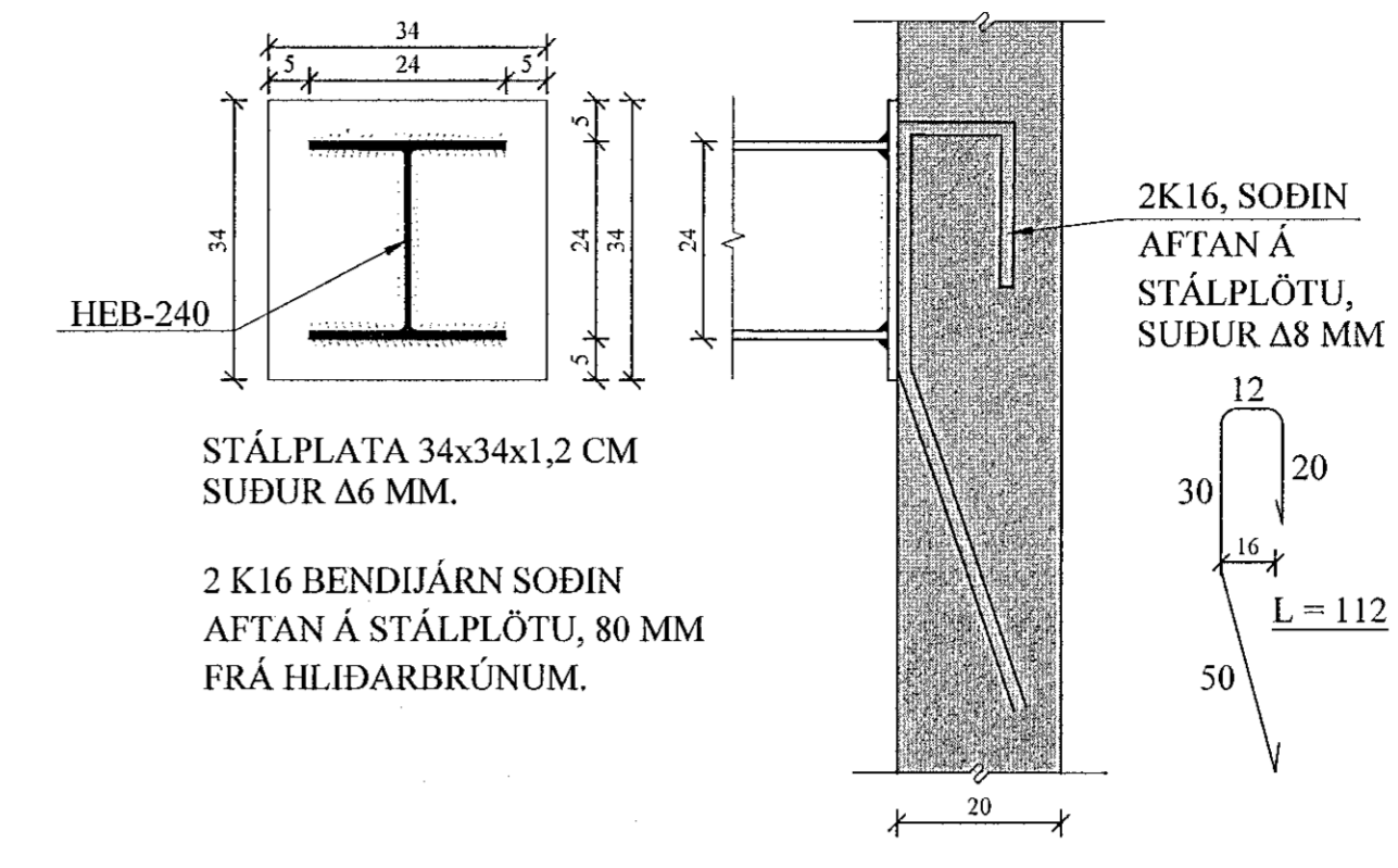
SM4 SÉRMYND. 1:10 1-11
