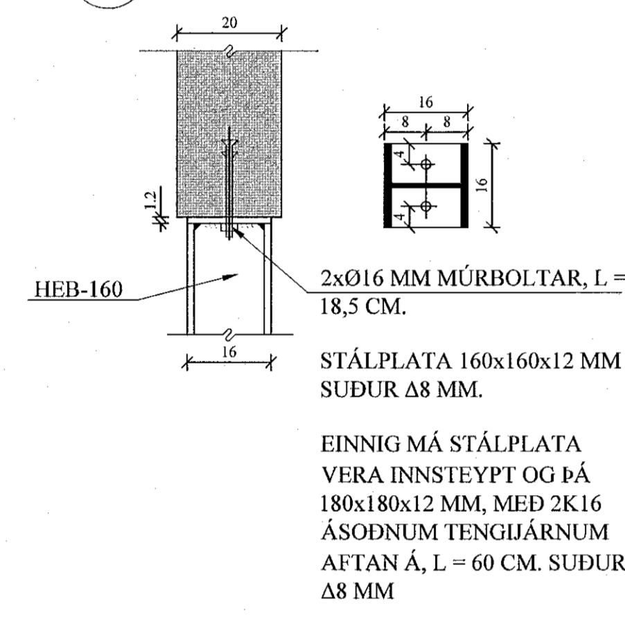
SM5 SÉRMYND. 1:10 1-11
