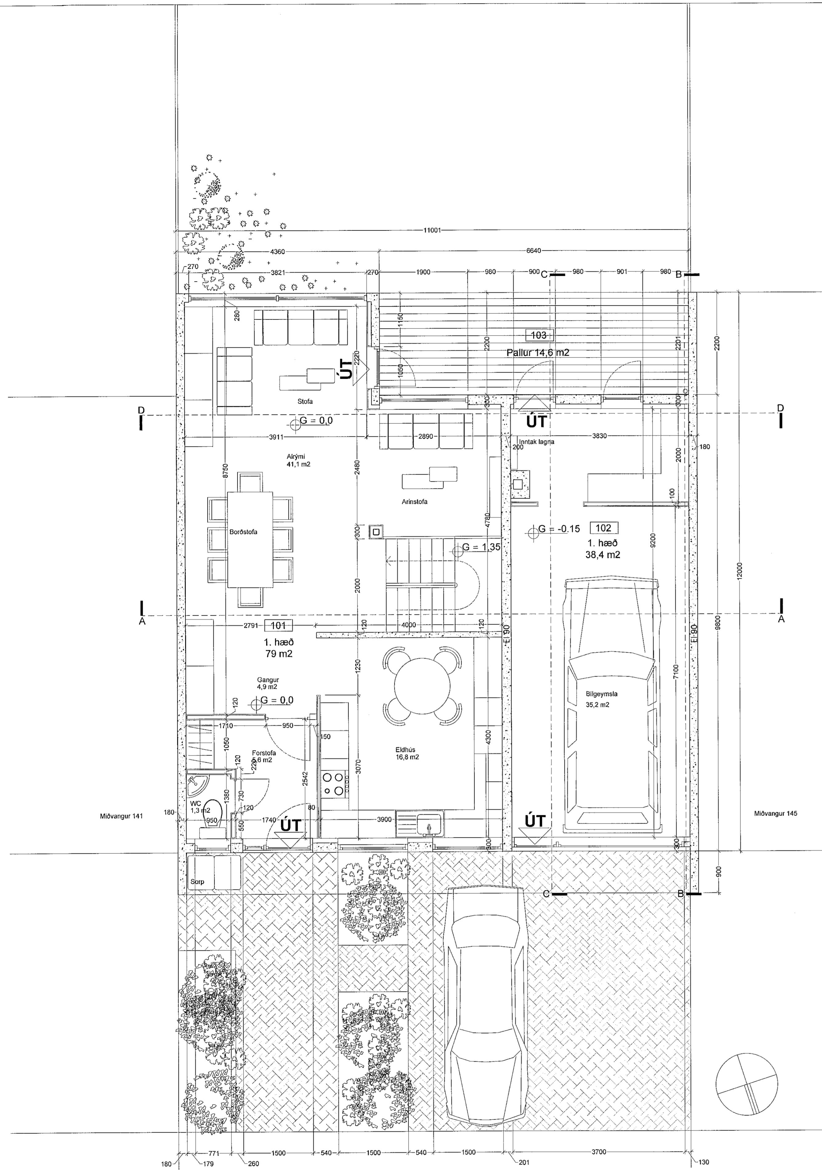
1 Grunnmynd jarðhæðar Mkv. 1:50
