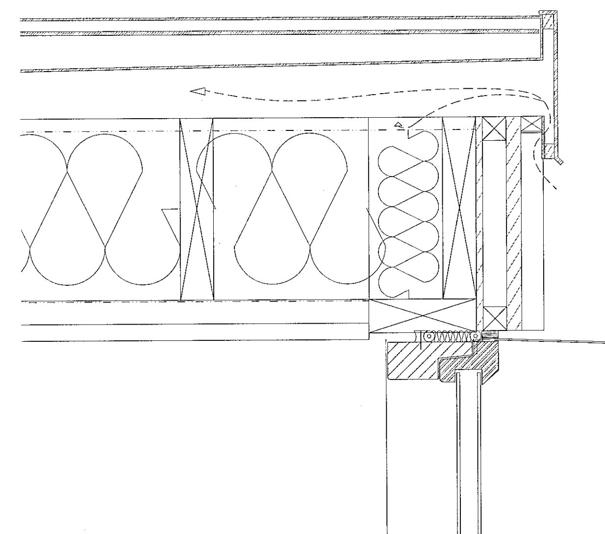
3 Lóðrétt deili V3.01 Mkv. 1:5
