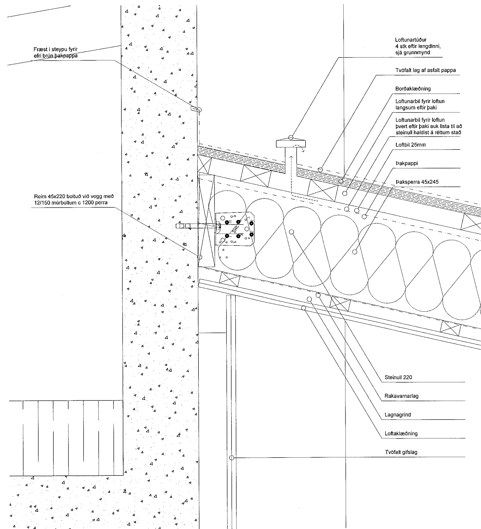
1 Lóðrétt deili V3.01 Mkv. 1:5
