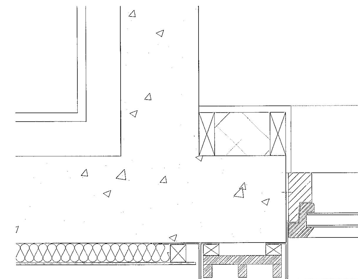
A Lárétt deili V3.01 Mkv. 1:5
