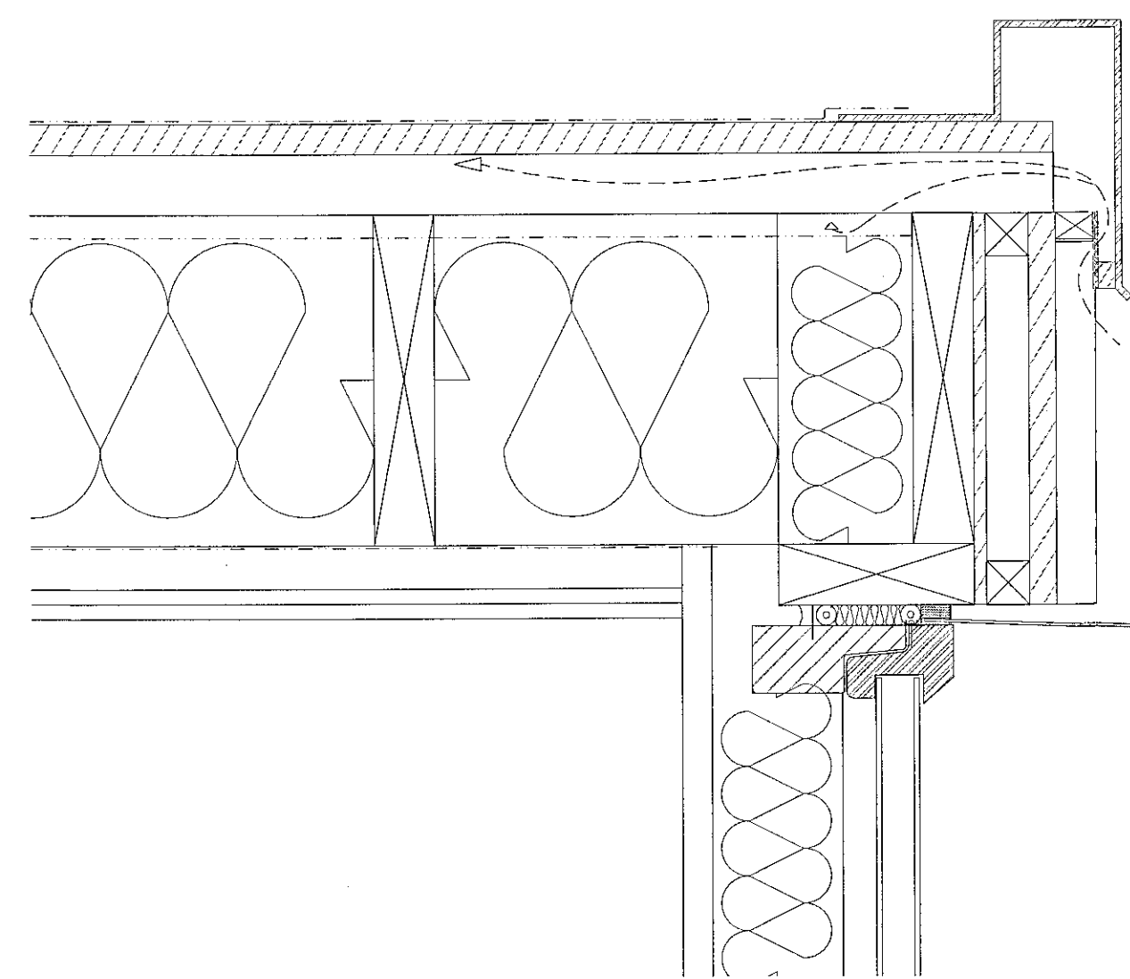
4 Lóðrétt deili V3.01 Mkv. 1:5
