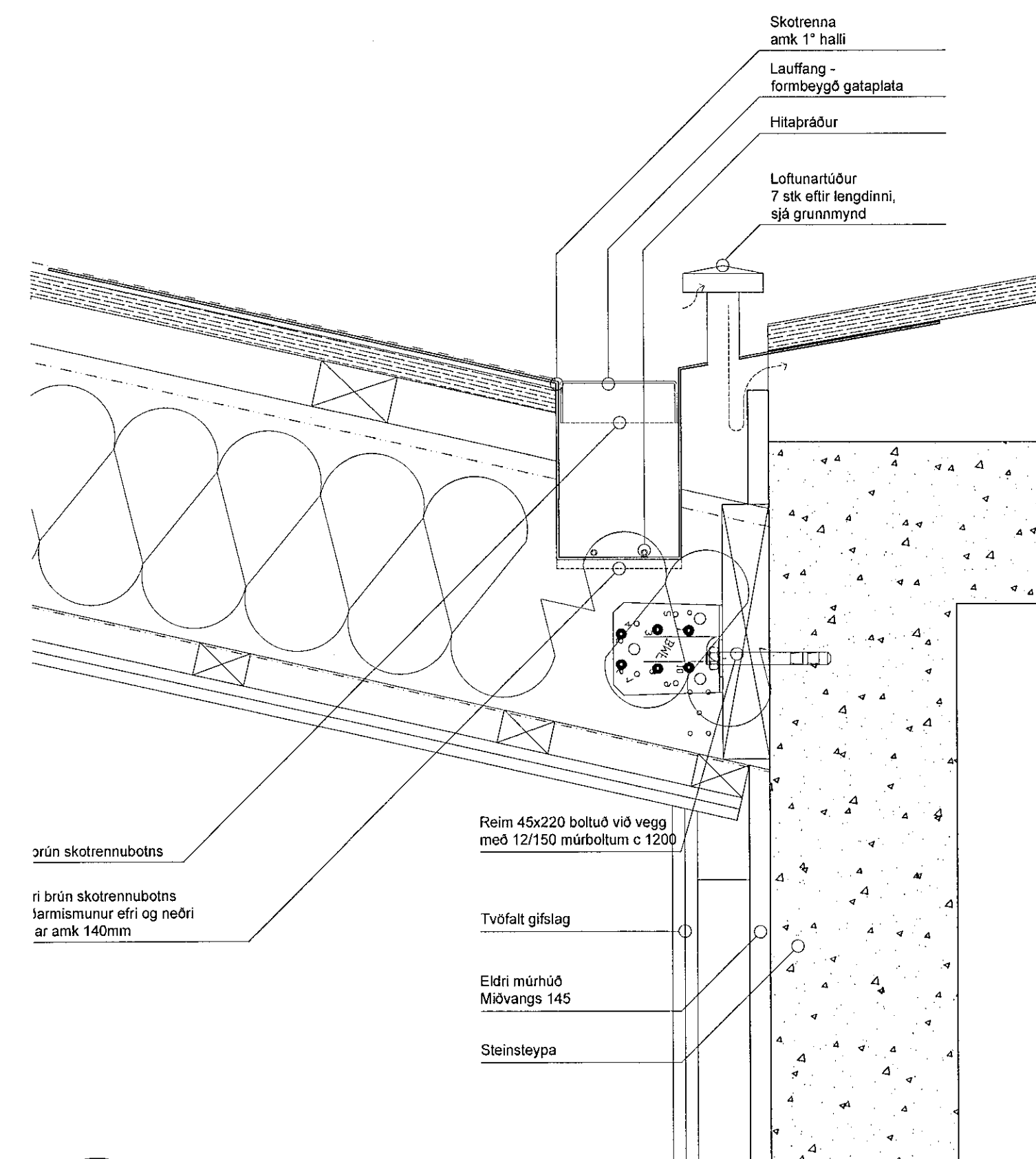
2 Lóðrétt deili V3.01 Mkv. 1:5
