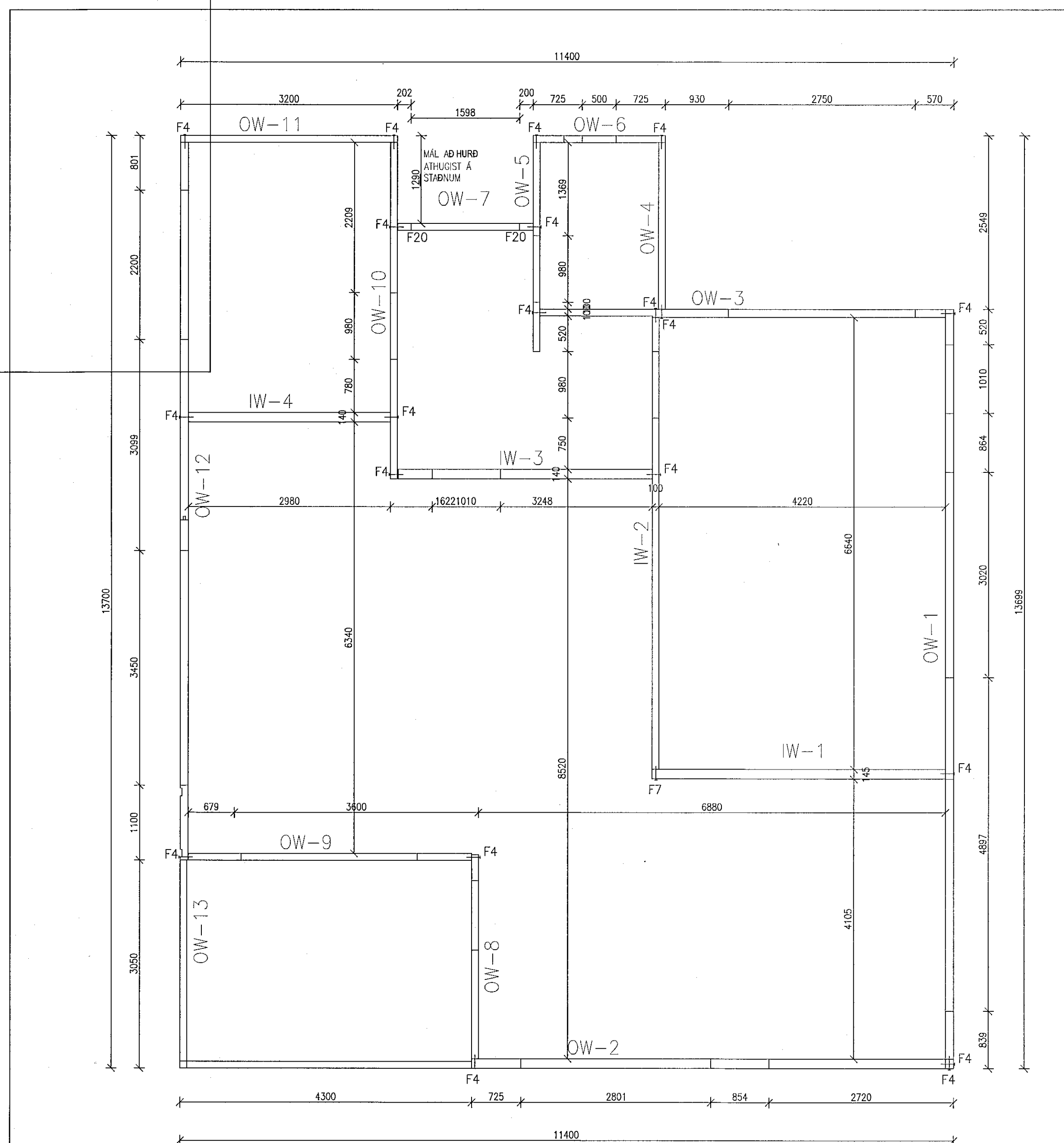
VEGGEININGAR 2. HÆÐ GRUNNMYND 1:50
