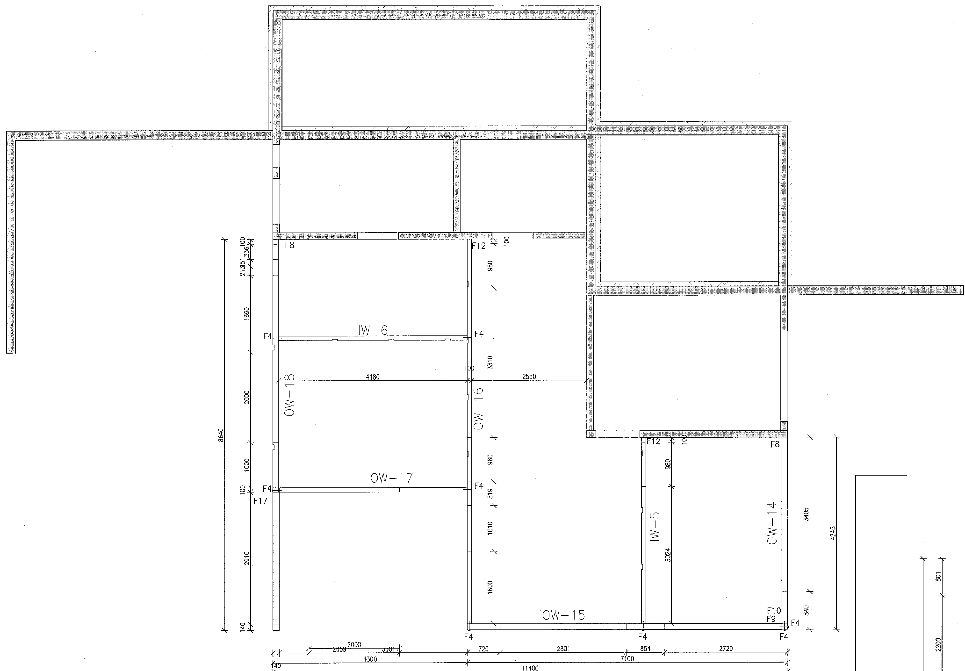
VEGGEININGAR 1. HÆÐ GRUNNMYND 1:50
