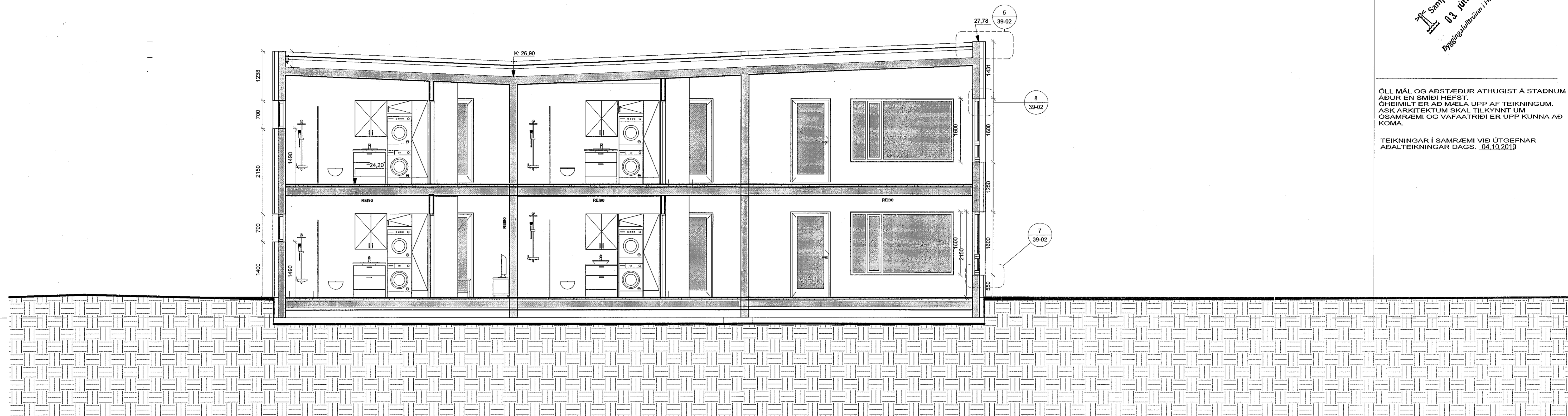
A-A Snið A-A snið 1 : 50
