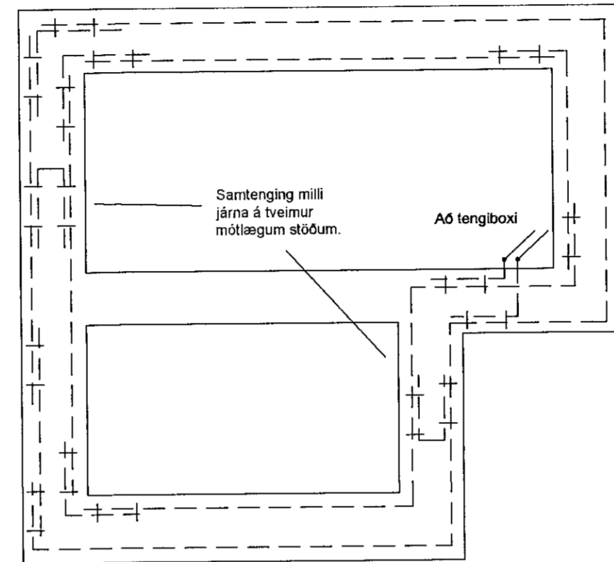
Gunnmynd sökkulveggja
