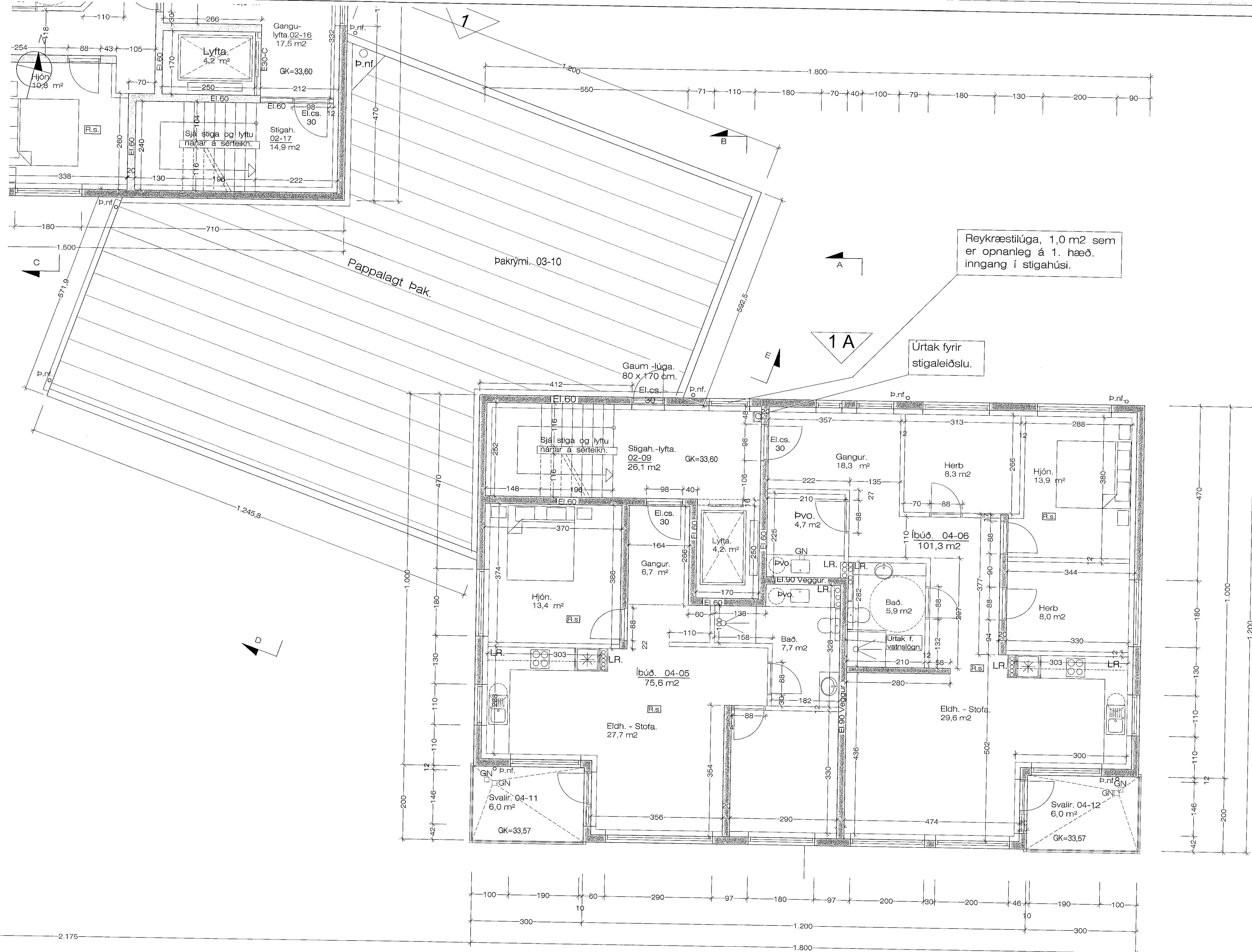
Grunnmynd 4. hæð. Hlutam. B. 1 : 50
