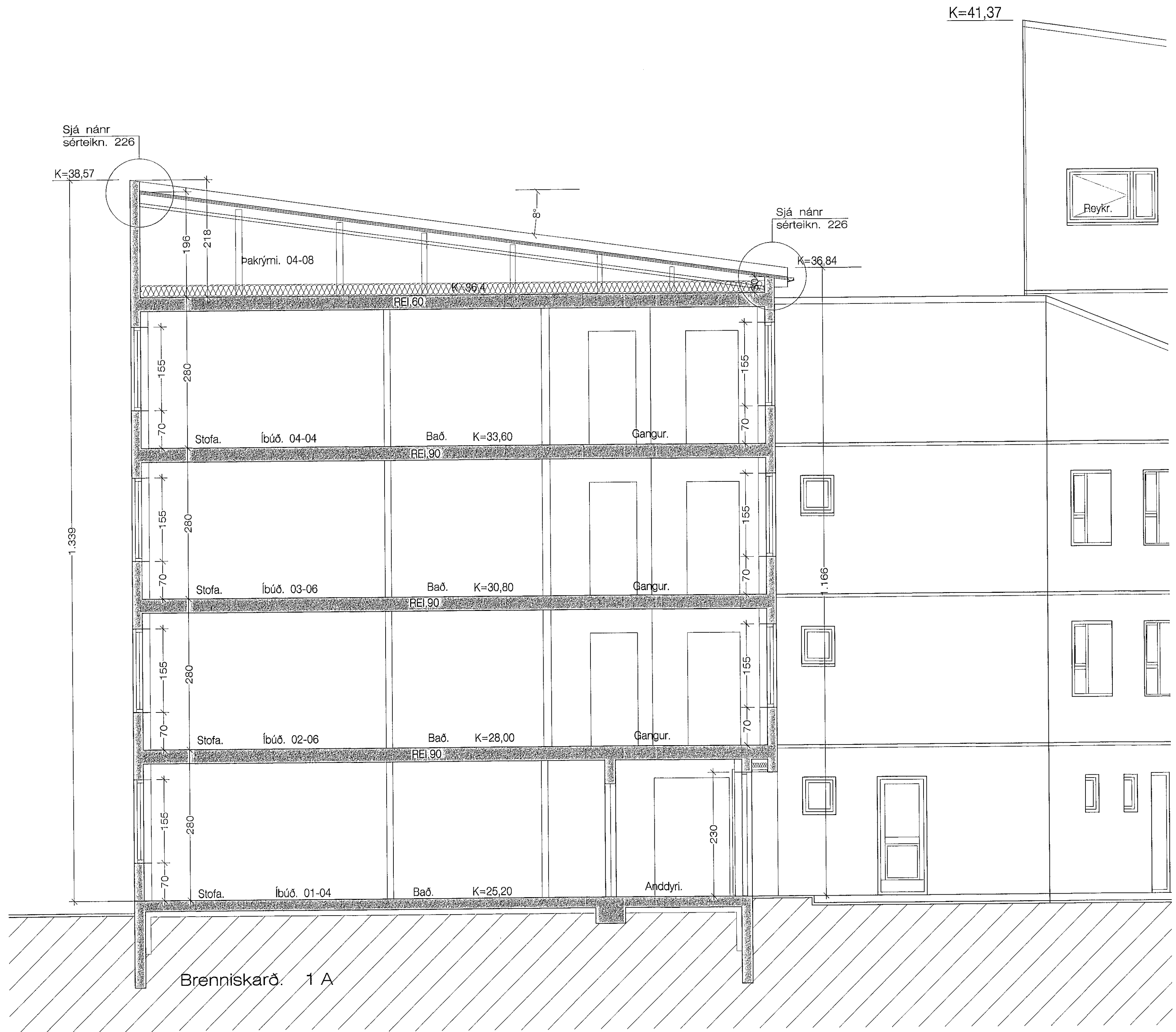
Sneiðing A - A 1 : 50
