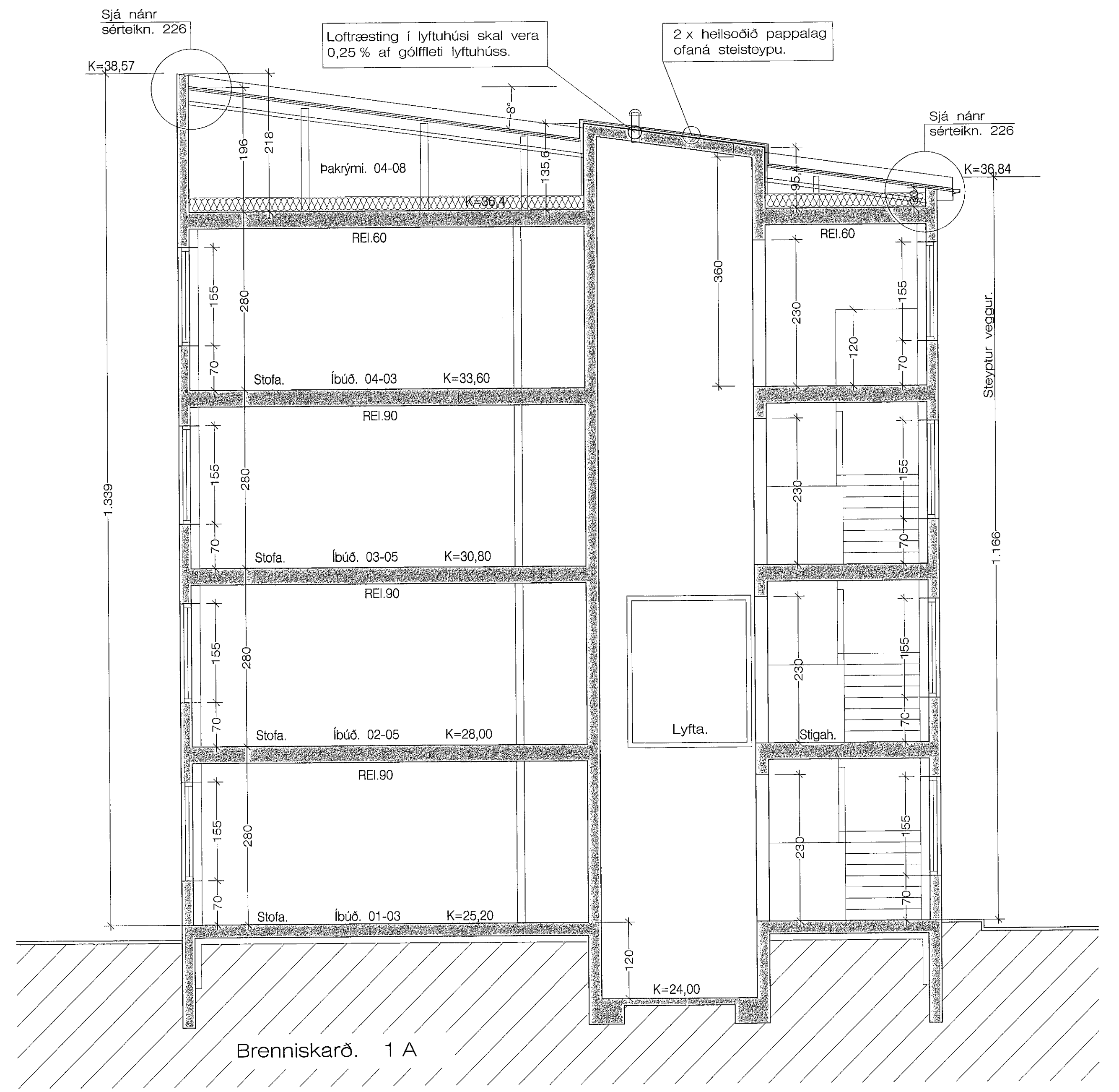
Sneiðing B - B 1 : 50
