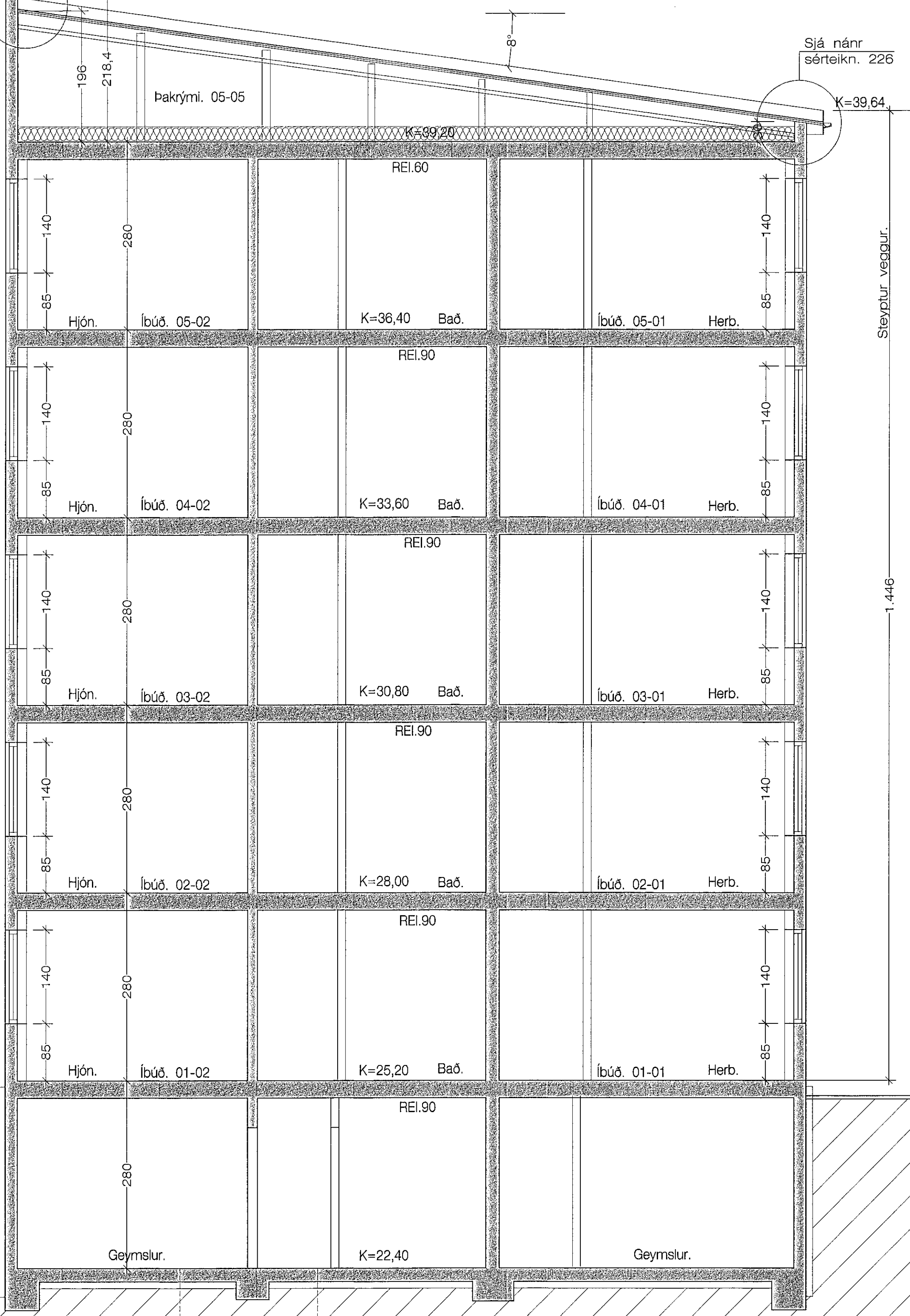
Sneiðing C - C 1 : 50
