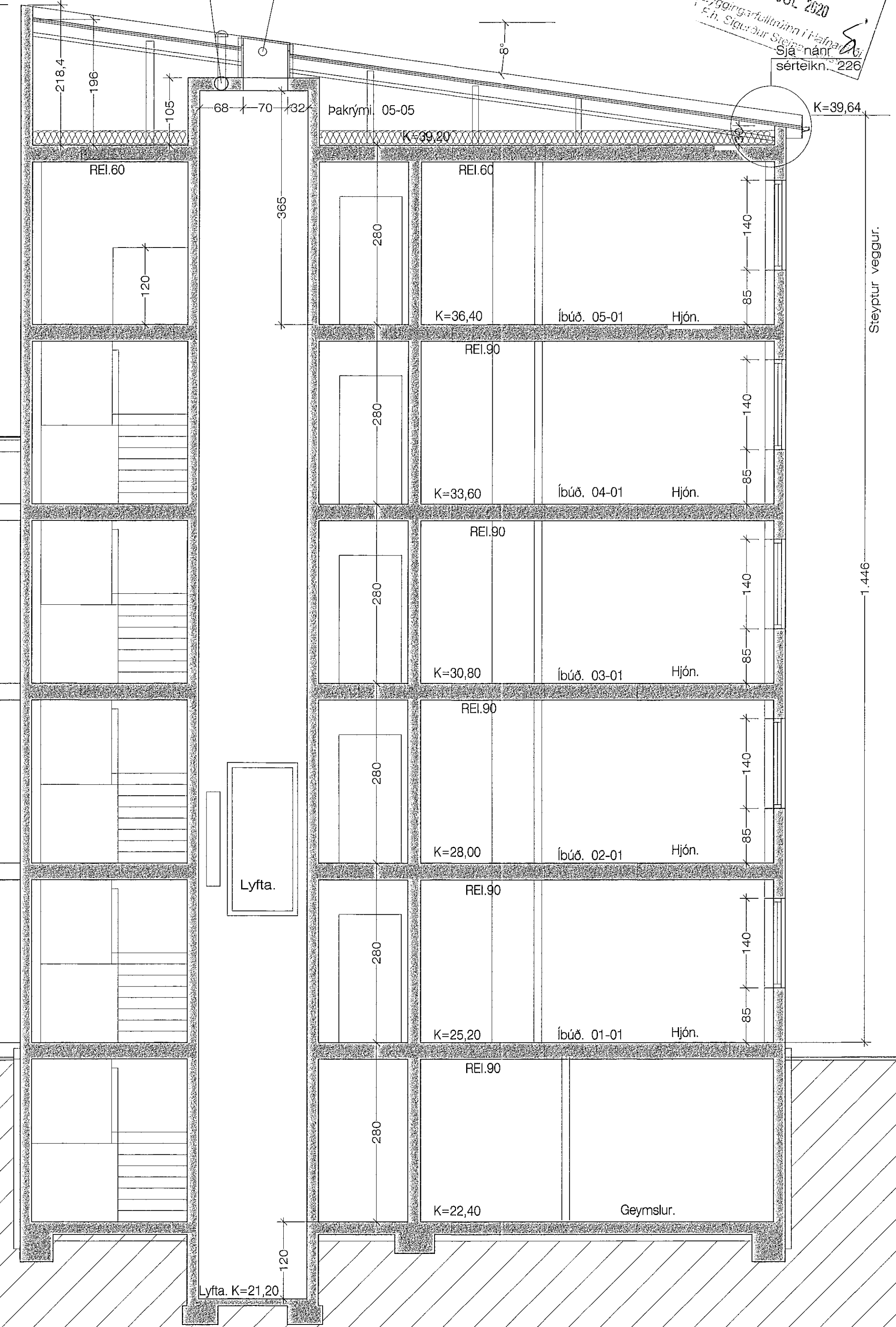
Sneiðing F - F 1 : 50
