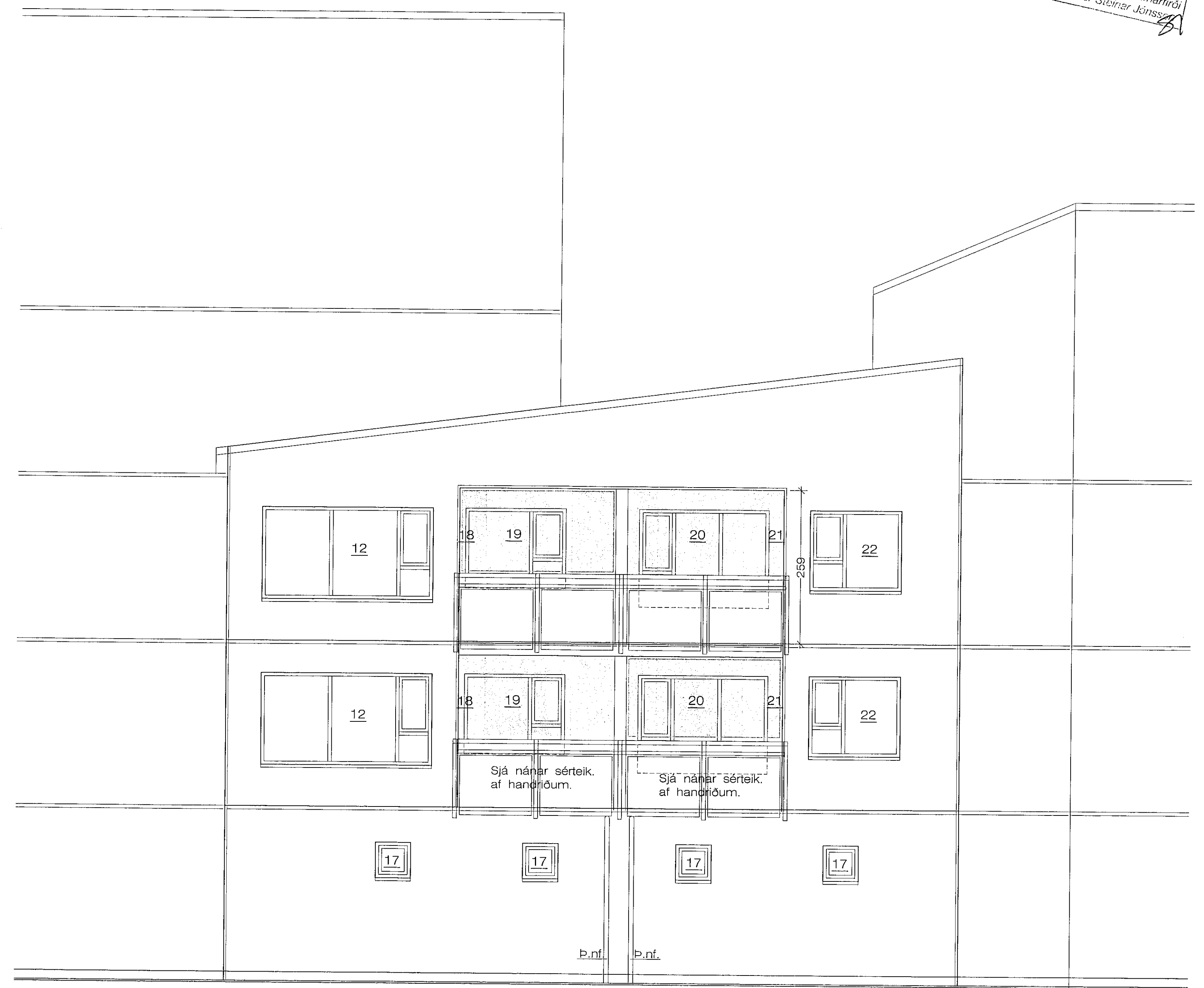
Suðurhlíð. Millibygging. 1 : 50 beint framaná hliðina.
