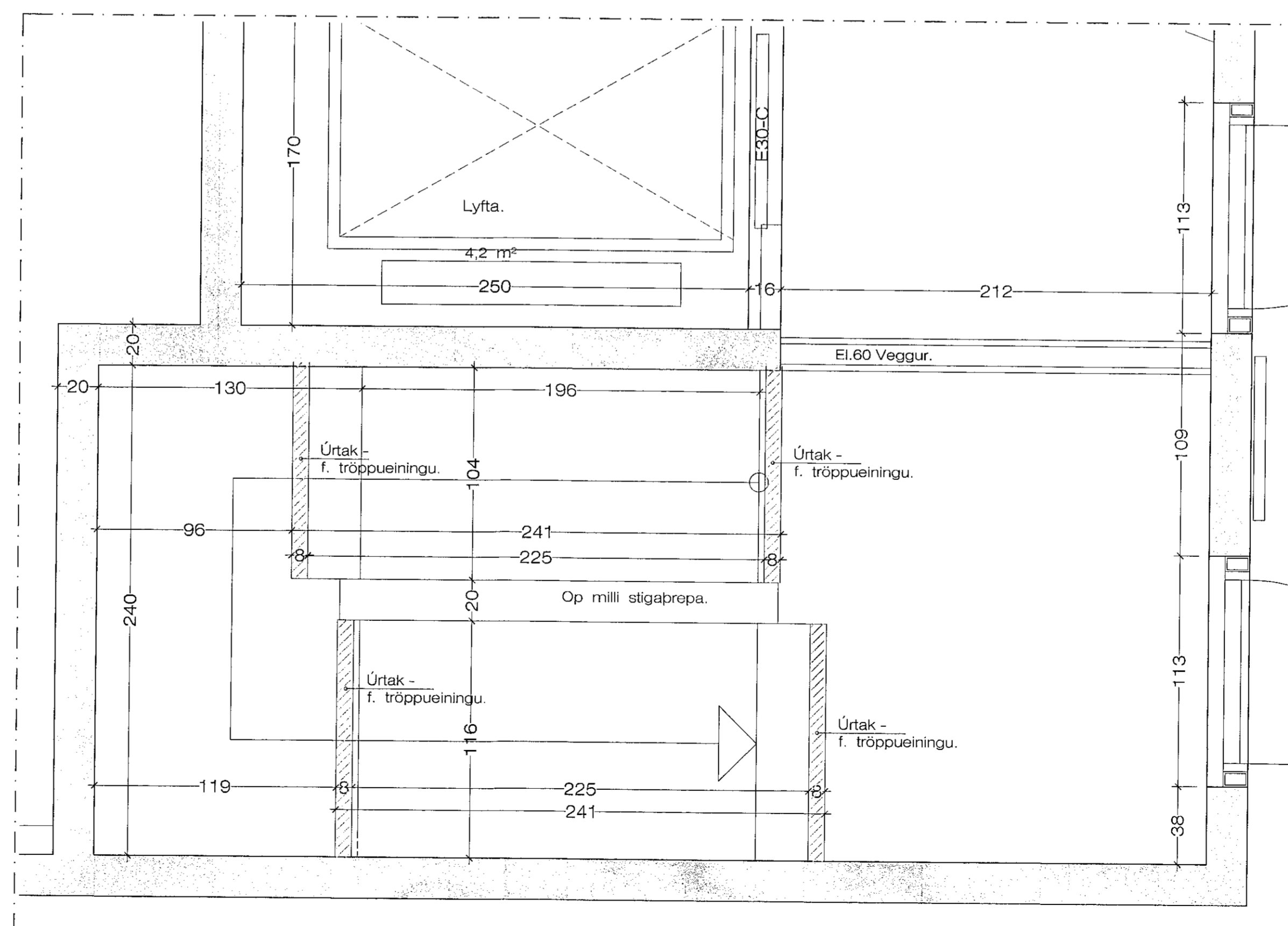
Úrtök fyrir tröppu einingar. 1:20
