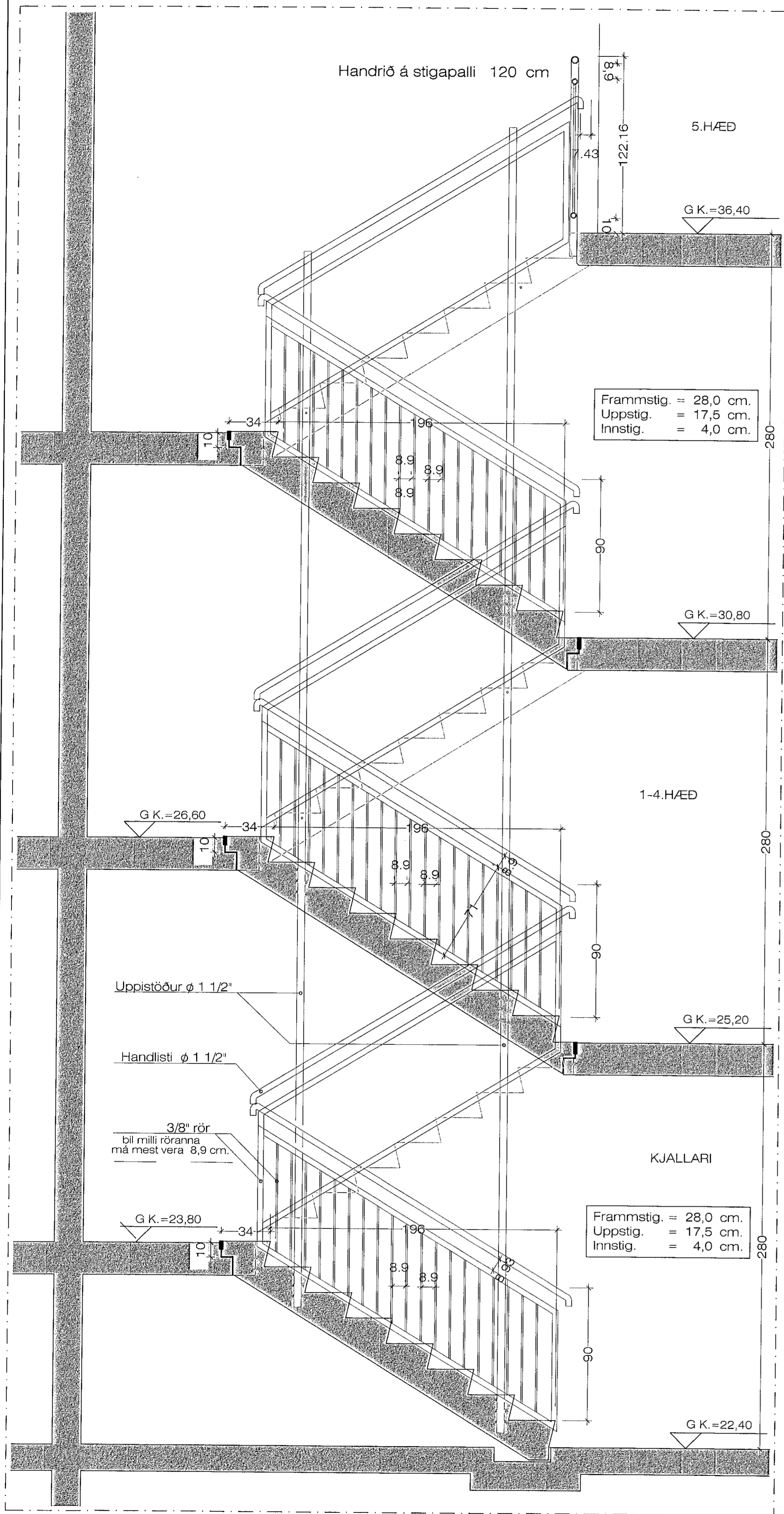
Sneiðing í stigahús. 1:20
