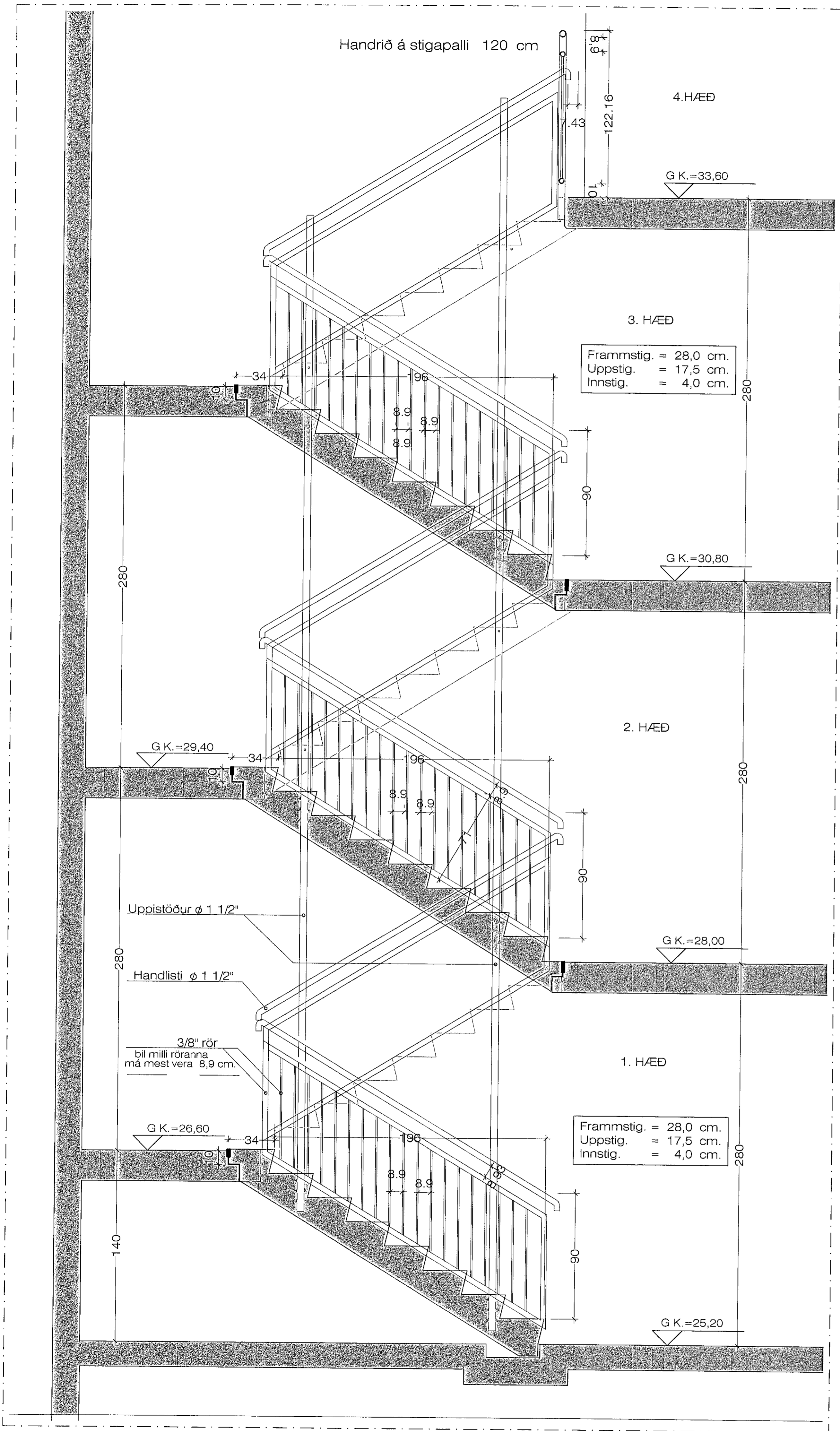
Sneiðing í stíga húsi. 1:20
