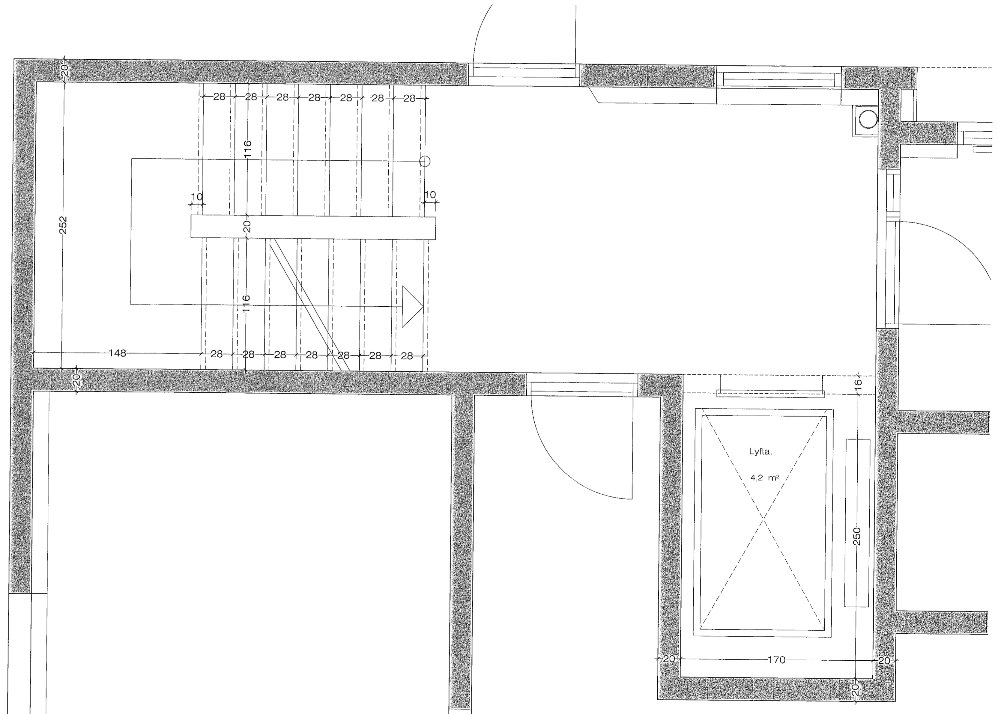
Grunnmynd af stíga húsi. 1:20
