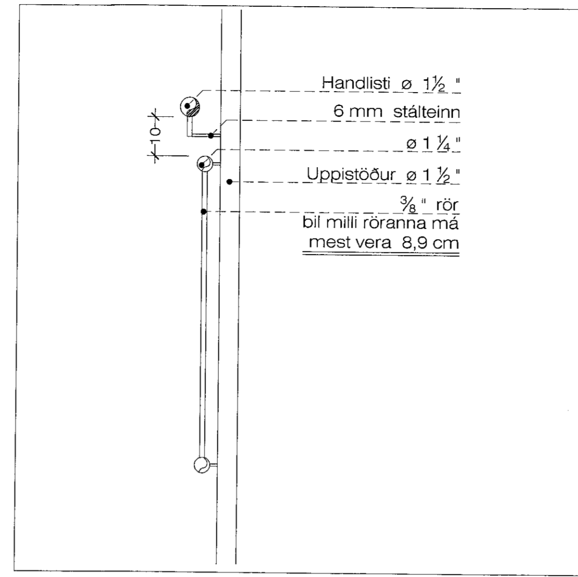
Handrið hlutamynd 1:10
